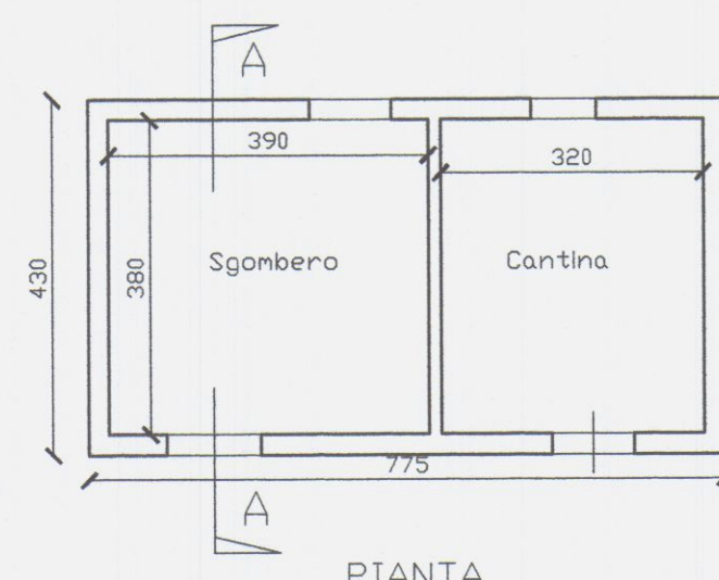
PIANTA
