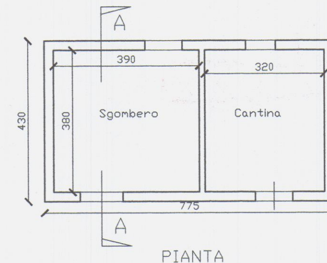
PIANTA
