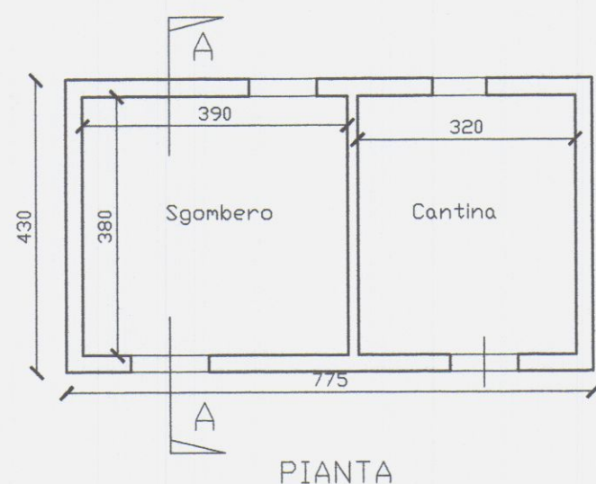
PIANTA
