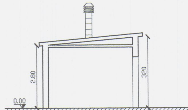
SEZIONE A-A
