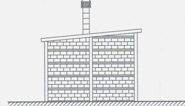
PROSPETTO EST
