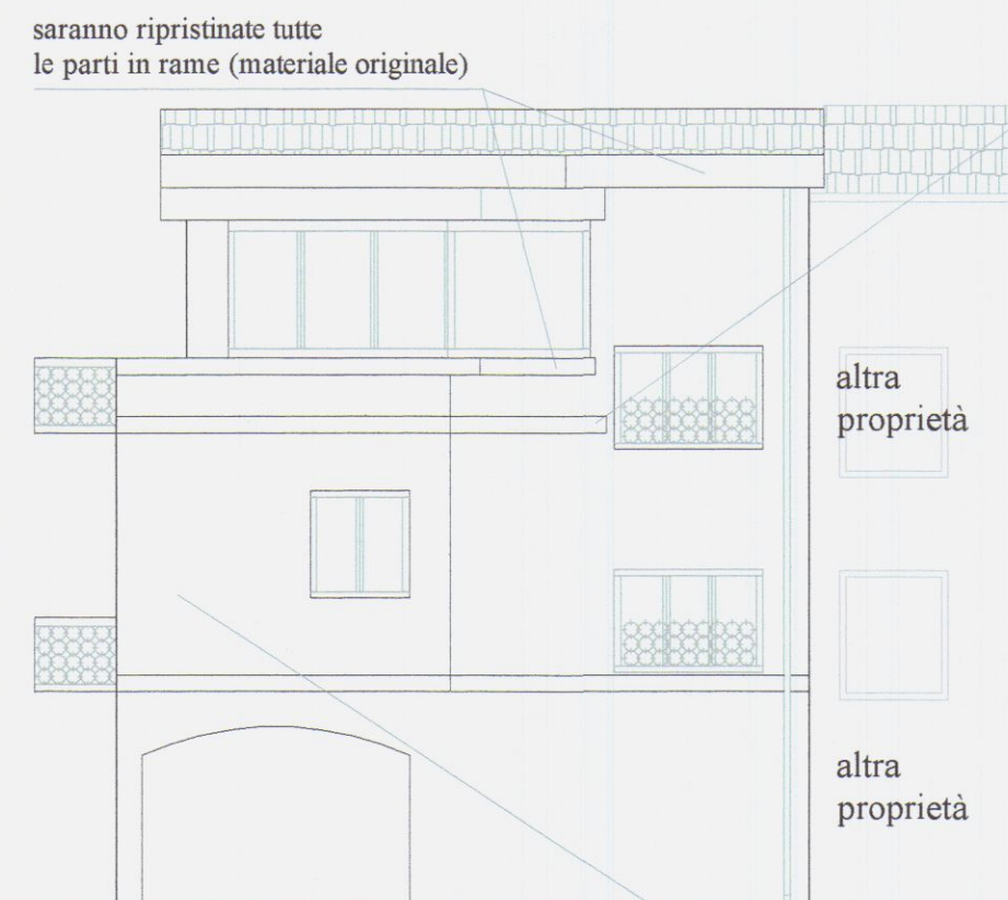
PROSPETTO NORD
