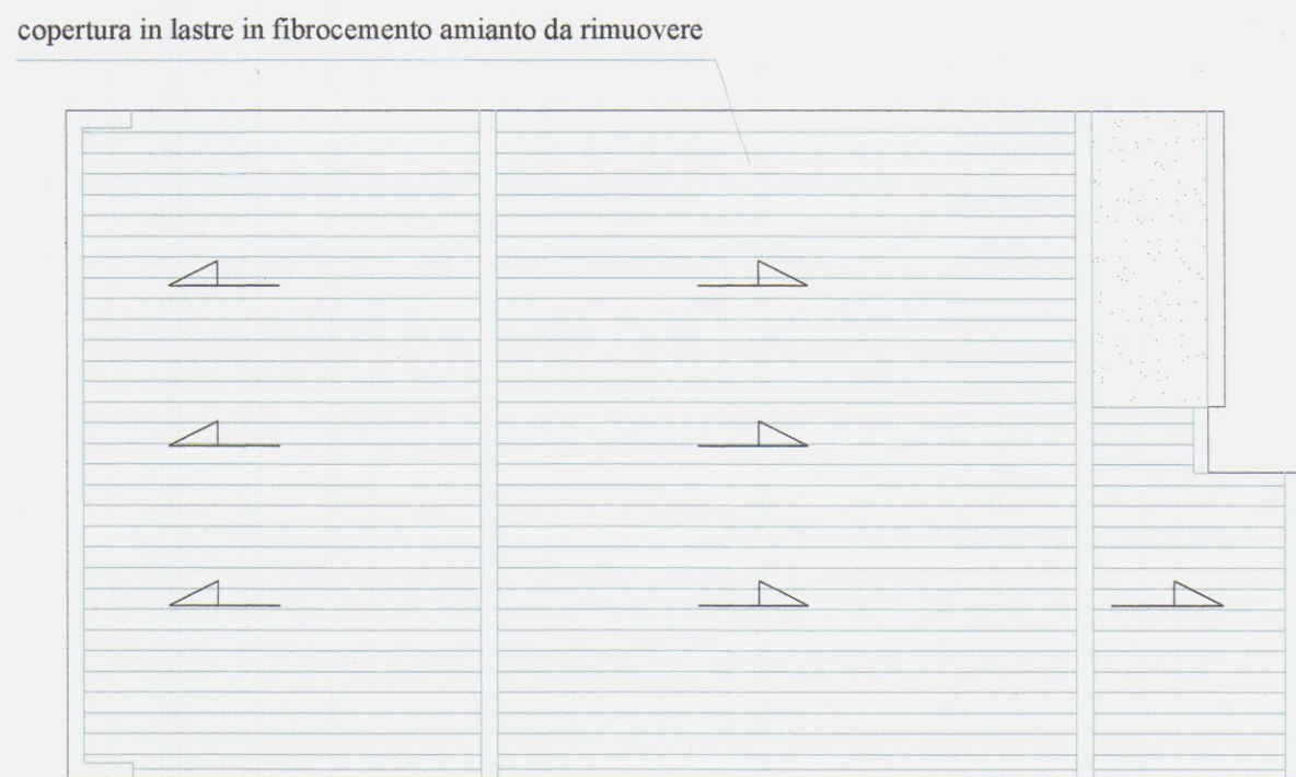
PIANTA COPERTURA
