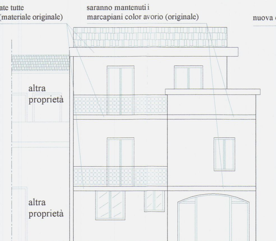
PROSPETTO SUD
