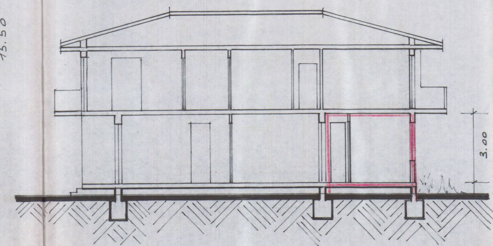
SEZIONE S - S
