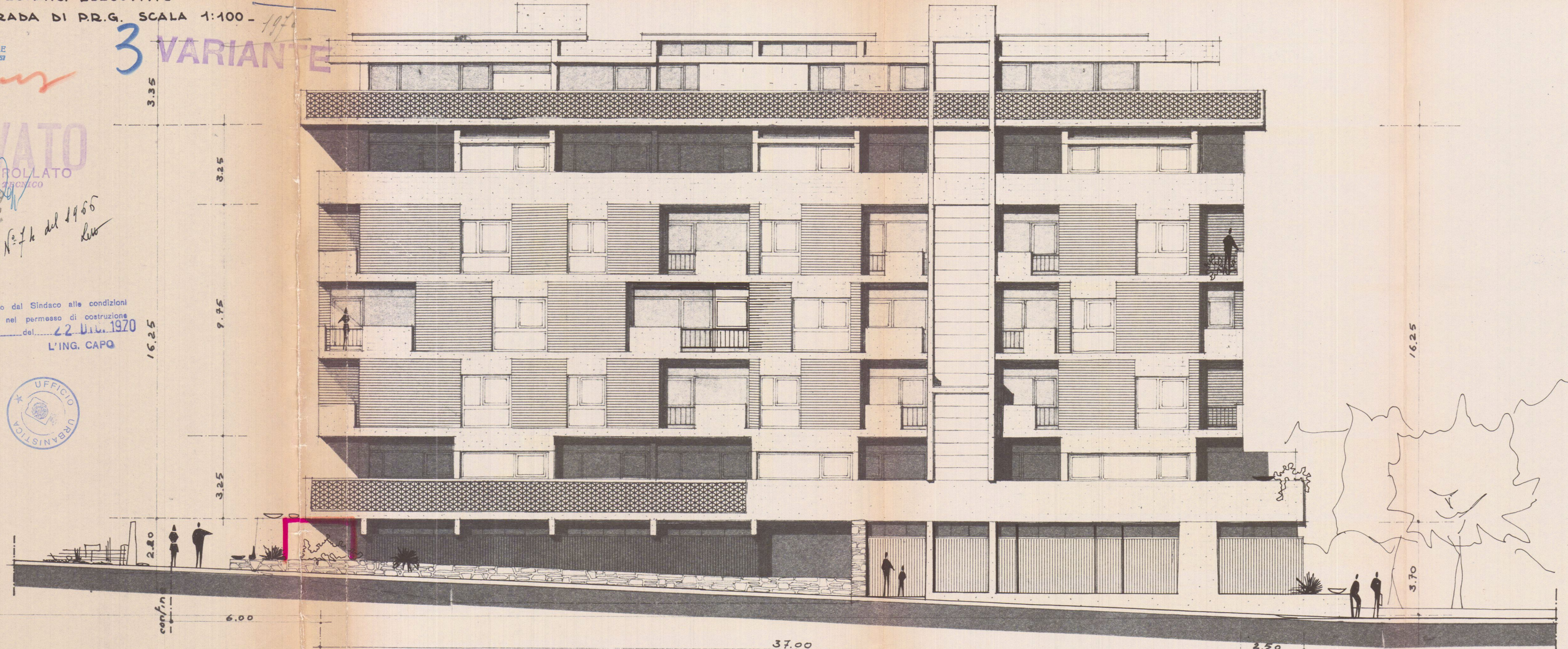
PROSPETTO SULLA VIA DI PENETRAZIONE 1:100 -
