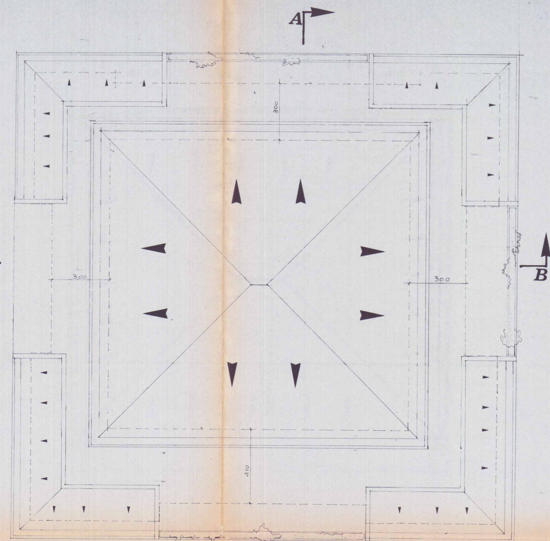
pianta copertura
