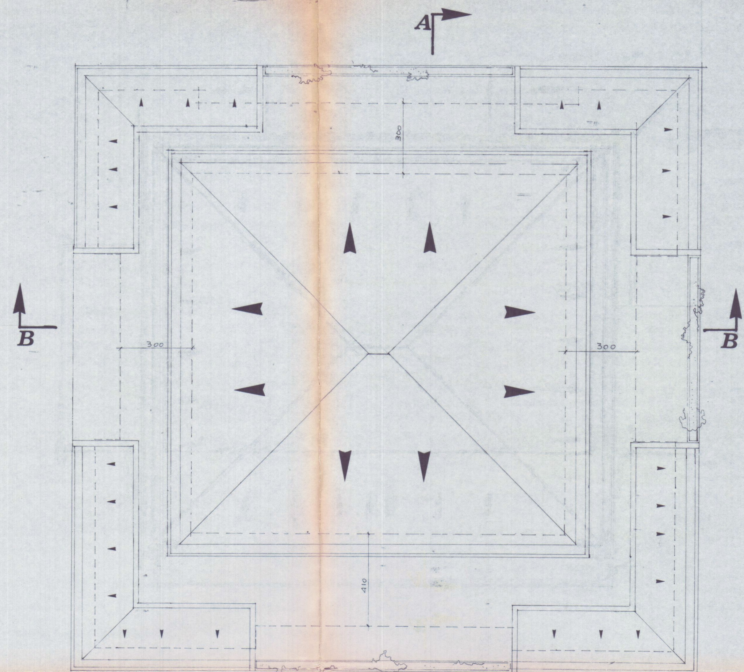
pianta copertura
