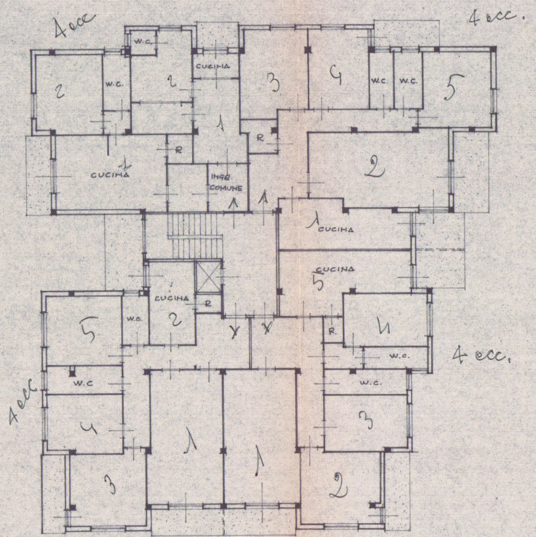
PIANO TERZO
