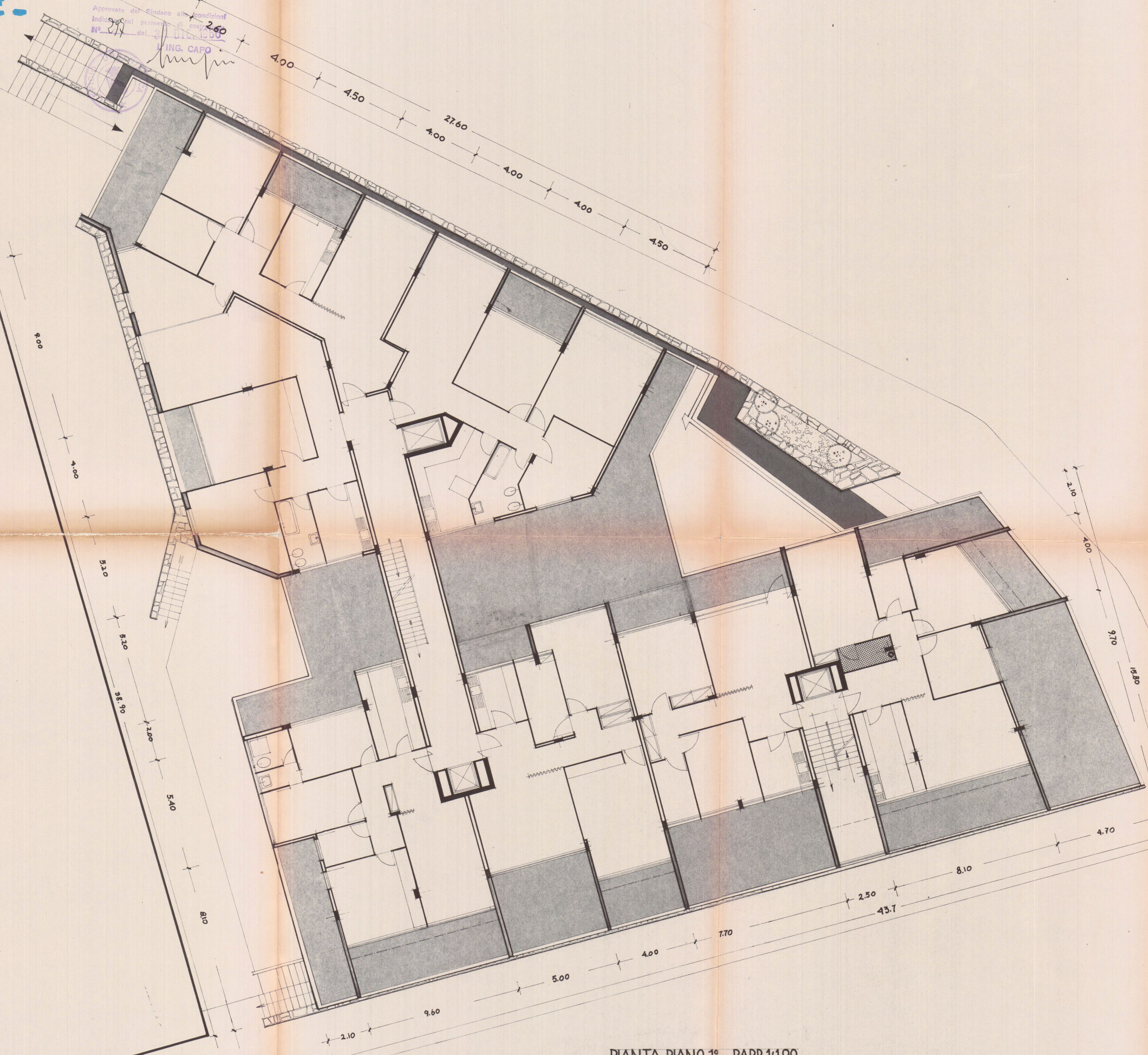
PIANTA PIANO 1° RAPR 1:100
