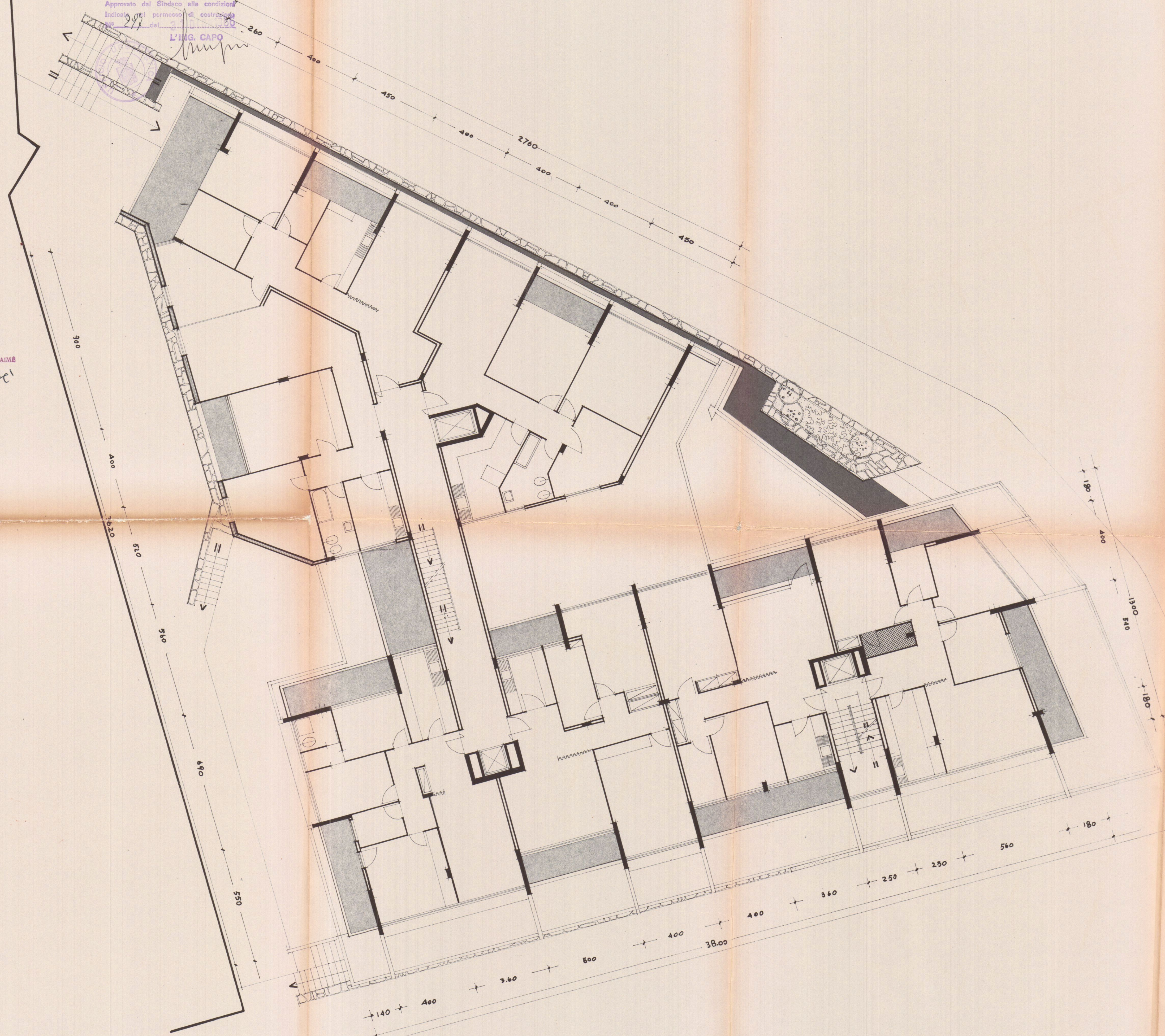
PIANTA PIANO 5° RAPP. 1:100
