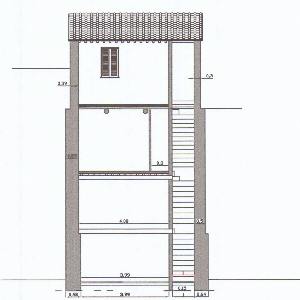
sezione C-C'
