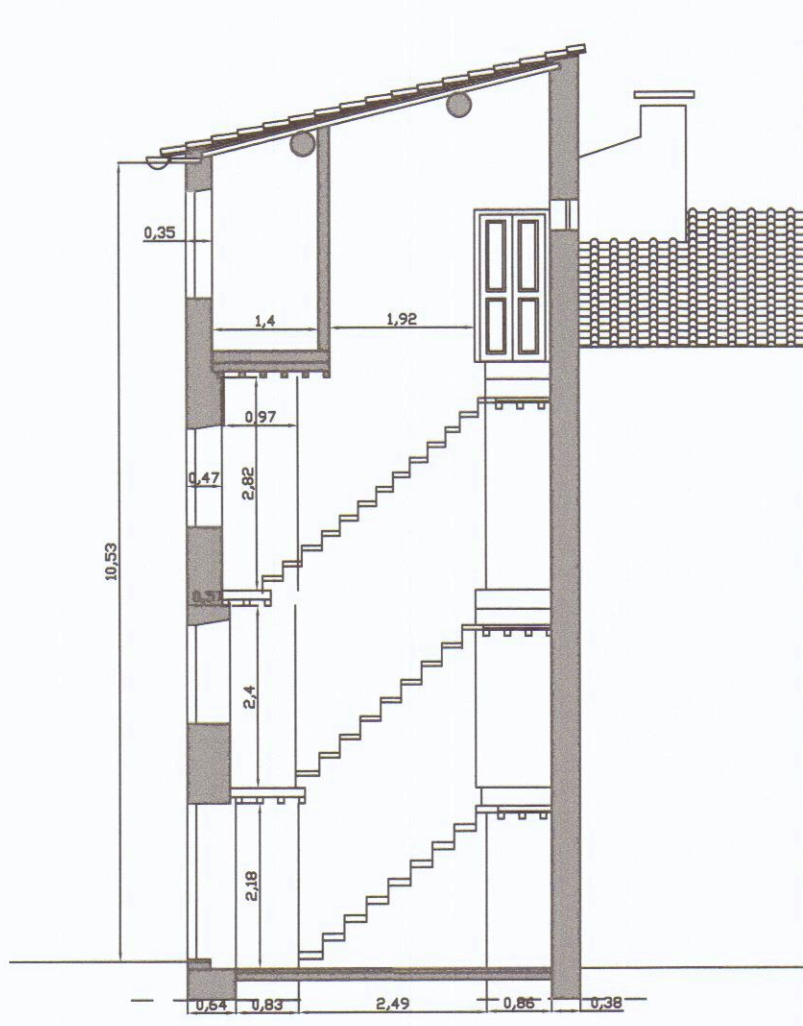
sezione A-A'
