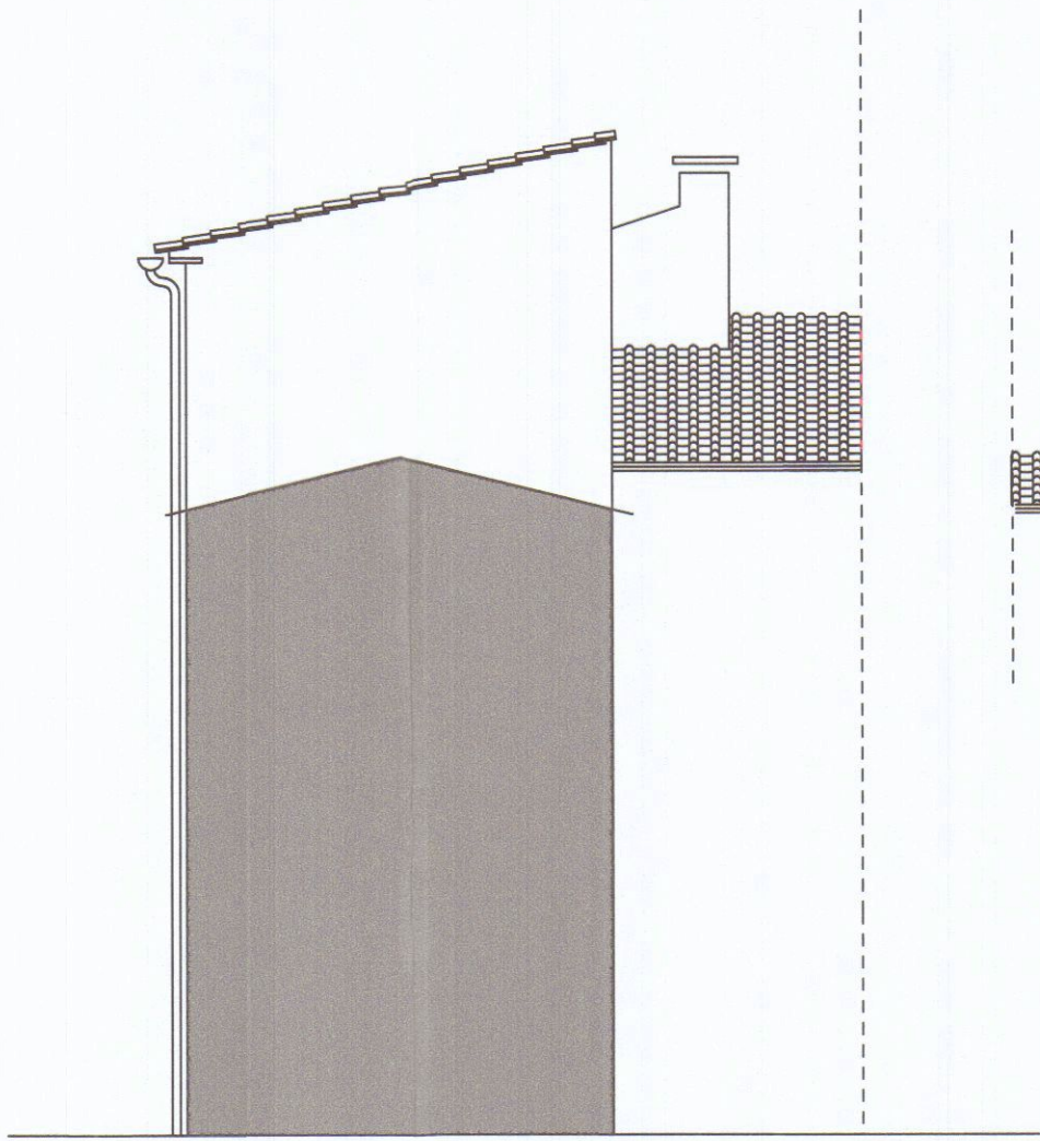
prospetto laterale
