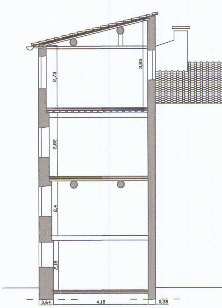
sezione B-B'
