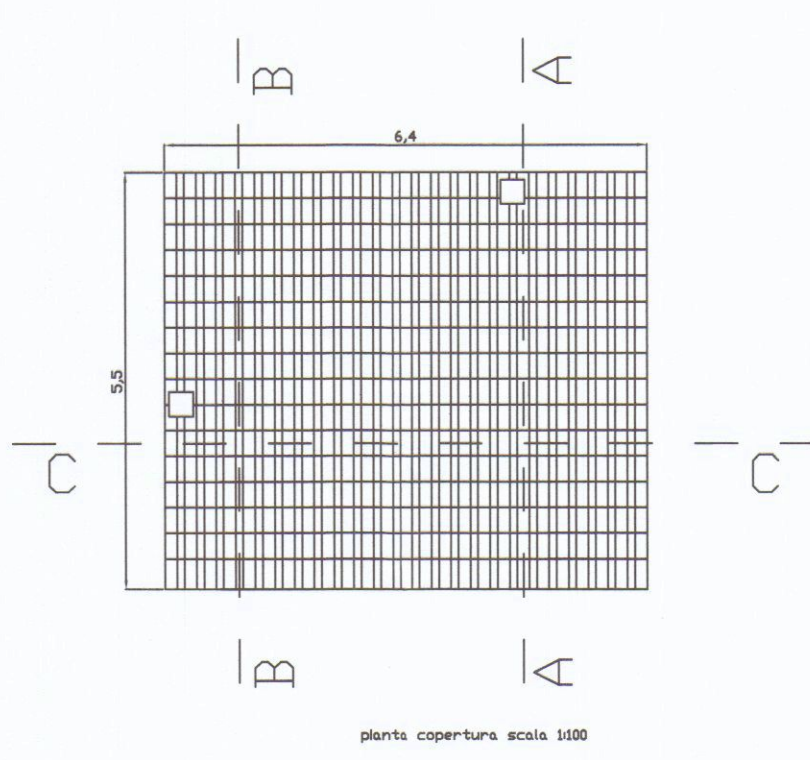
pianta copertura scala 1:100
