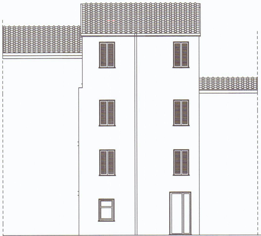
prospetto lato strada
