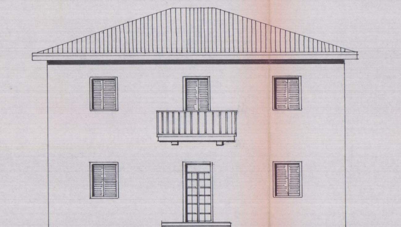
LATO SUD DA PROGETTO
