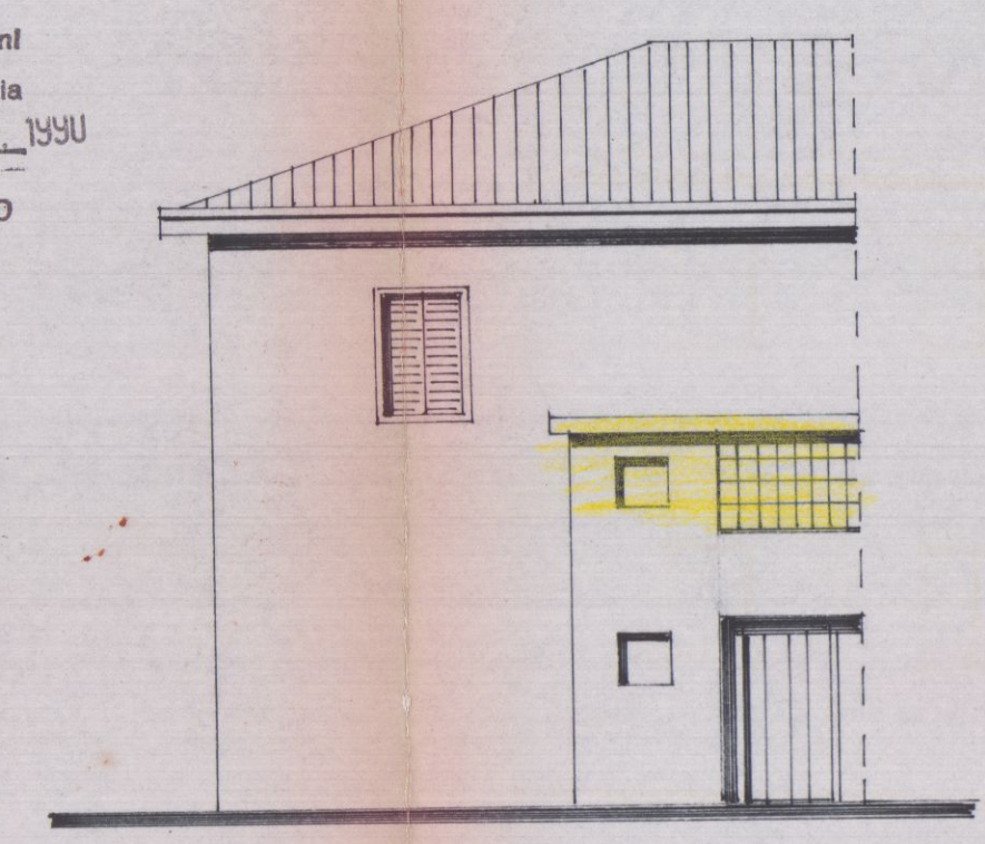
LATO NORD ESISTENTE
