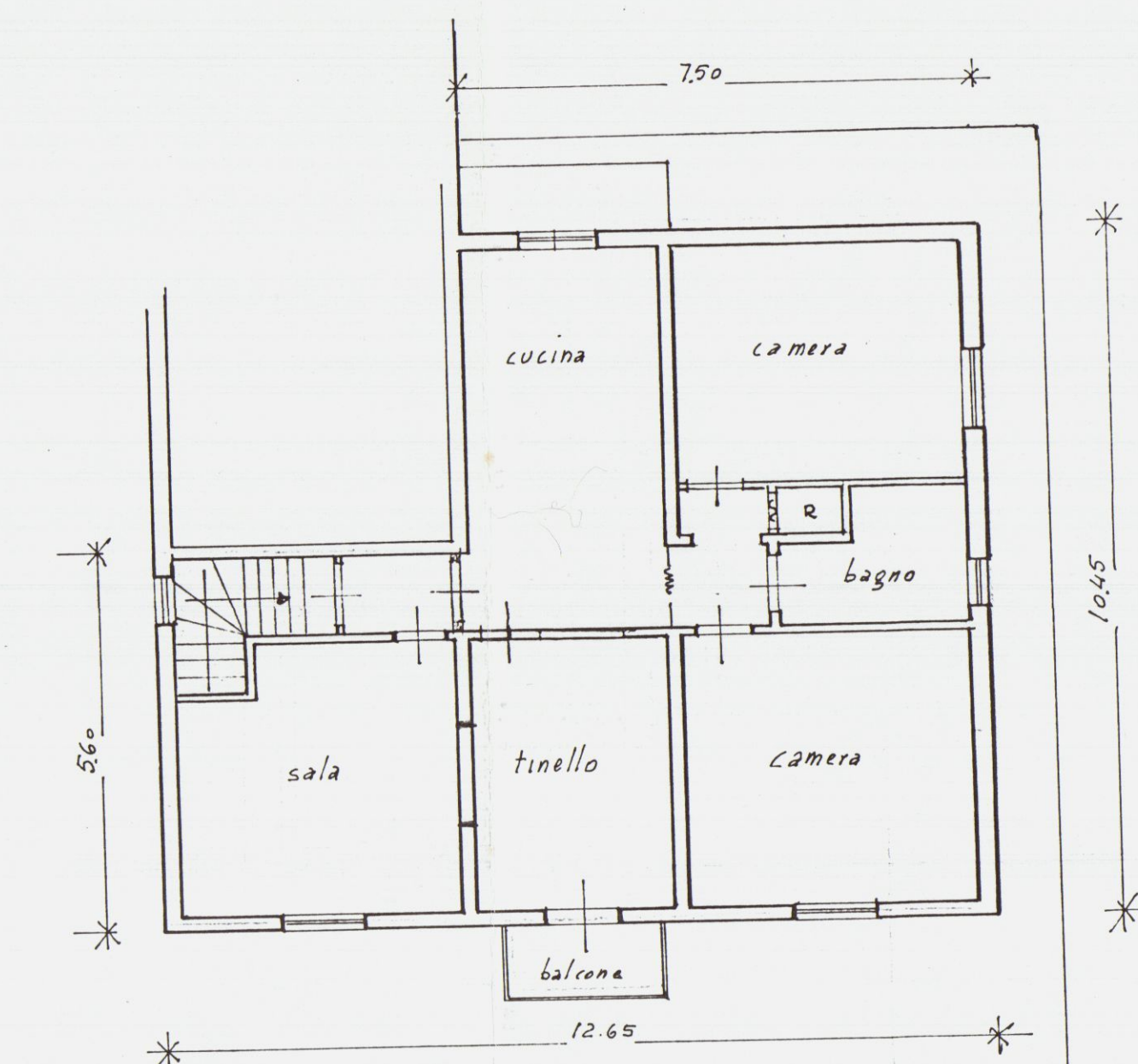
PIANO PRIMO DA PROGETTO
