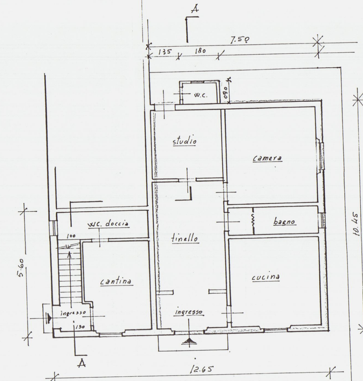
PIANOTERRA DA PROGETTO
