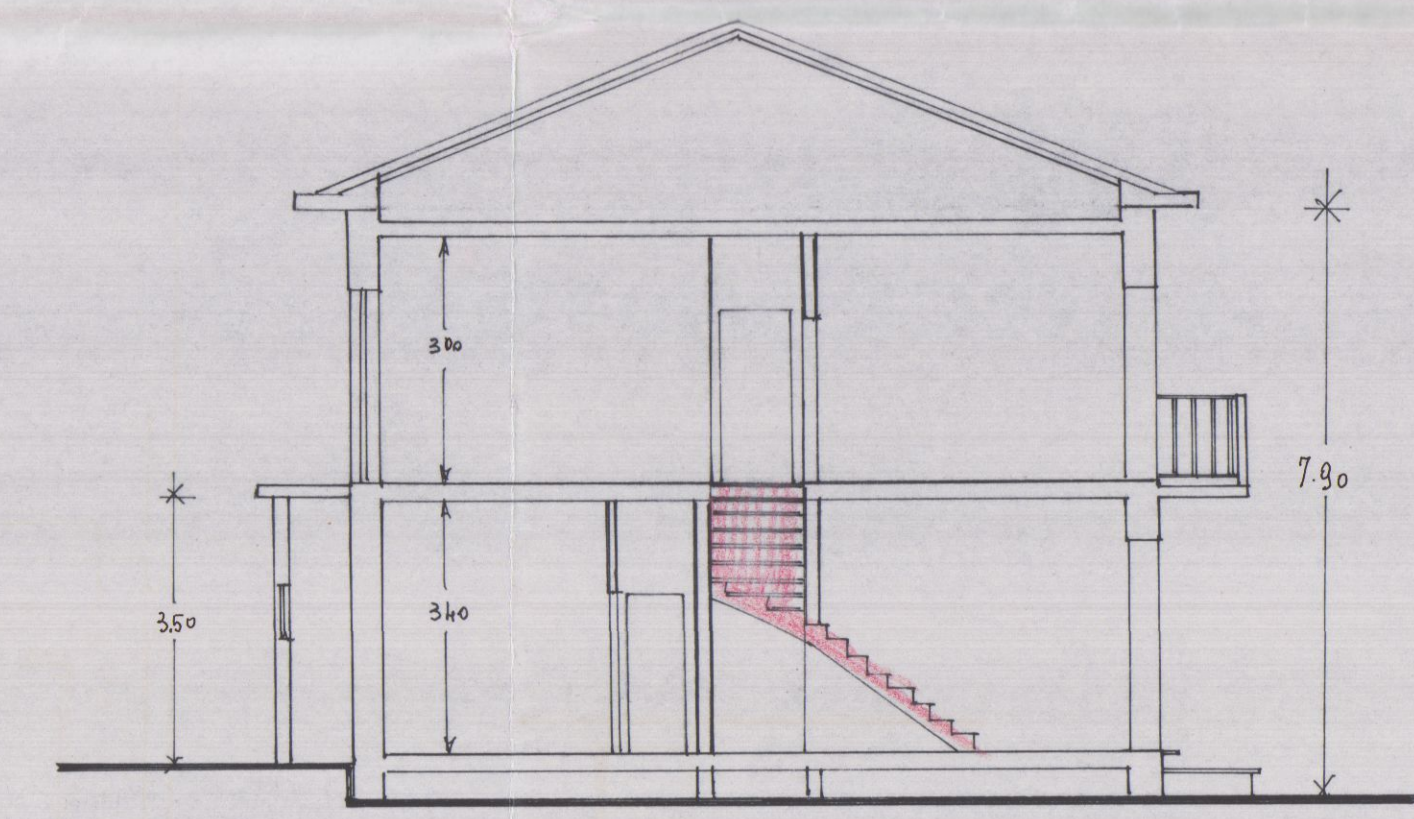
SEZIONE A-A DA PROGETTO
