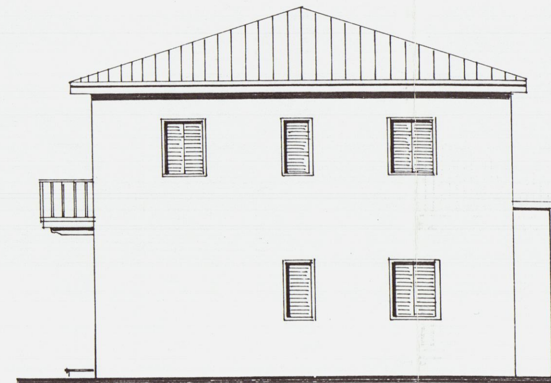
LATO EST ESISTENTE
