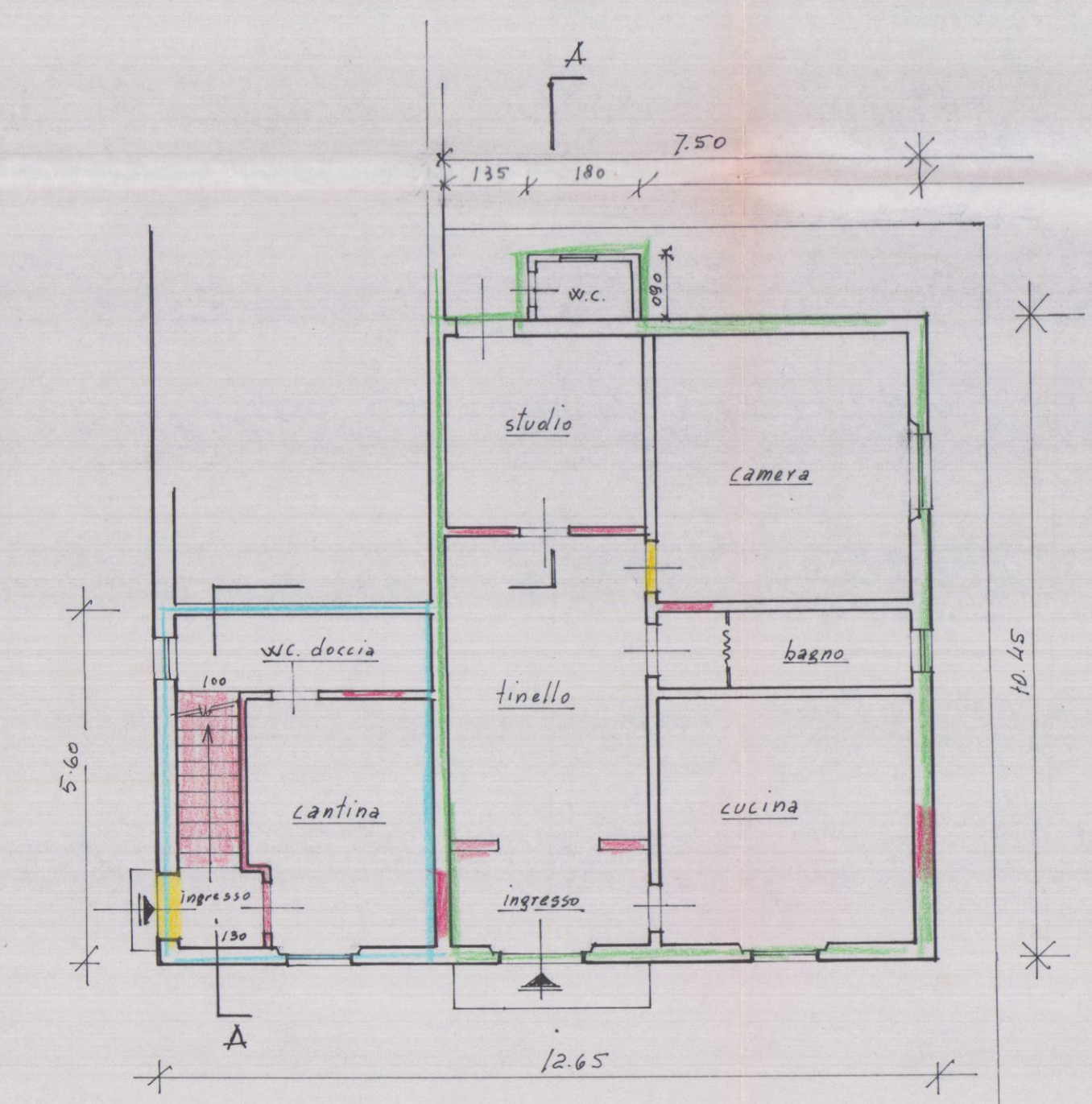
PIANOTERRA DA PROGETTO
