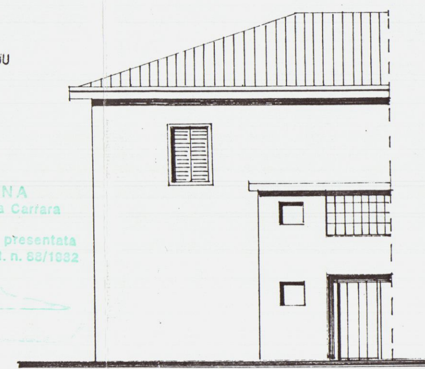
LATO NORD ESISTENTE
