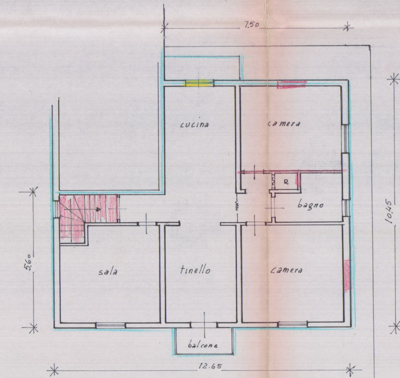
PIANO PRIMO DA PROGETTO
