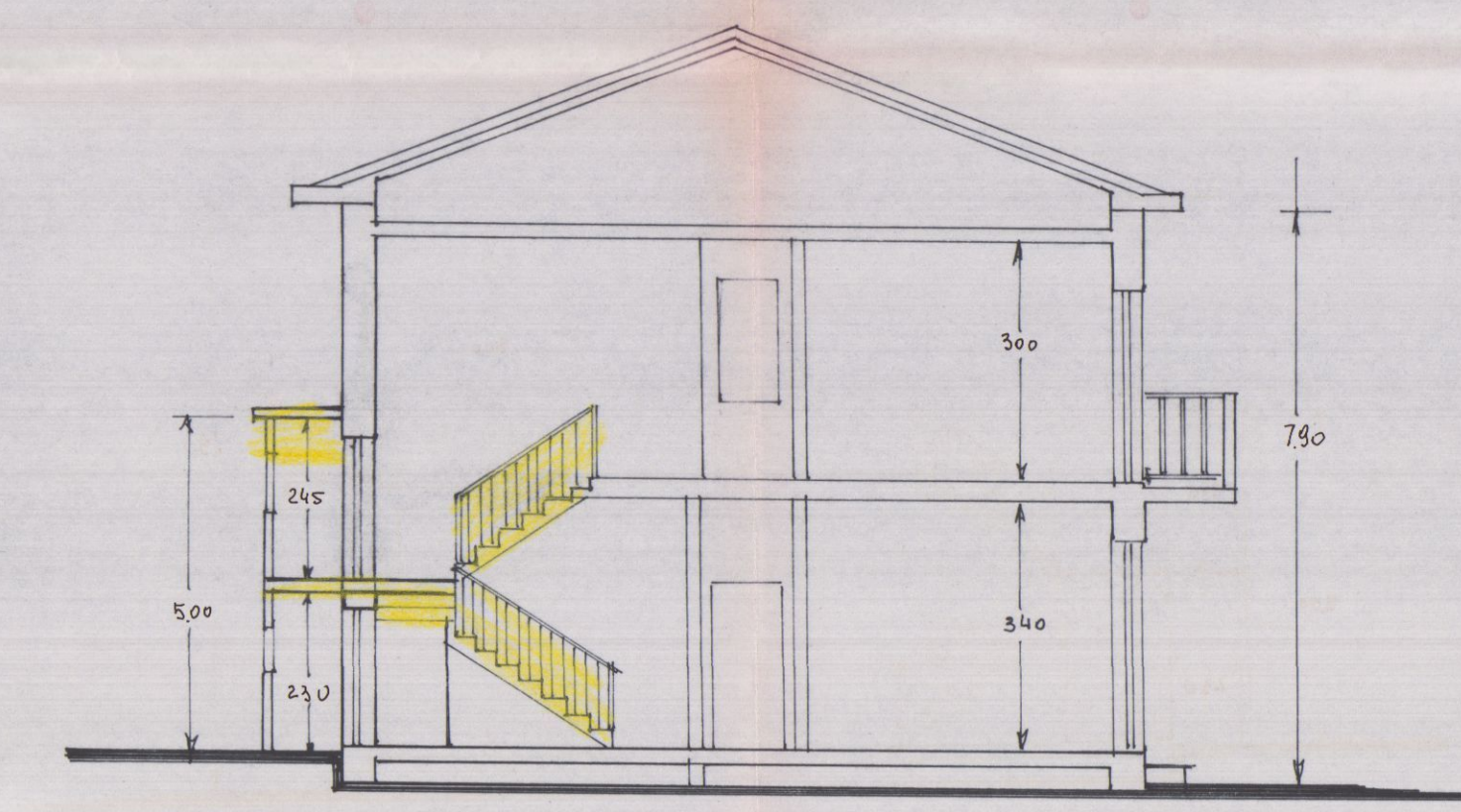
SEZIONE A-A ESISTENTE
