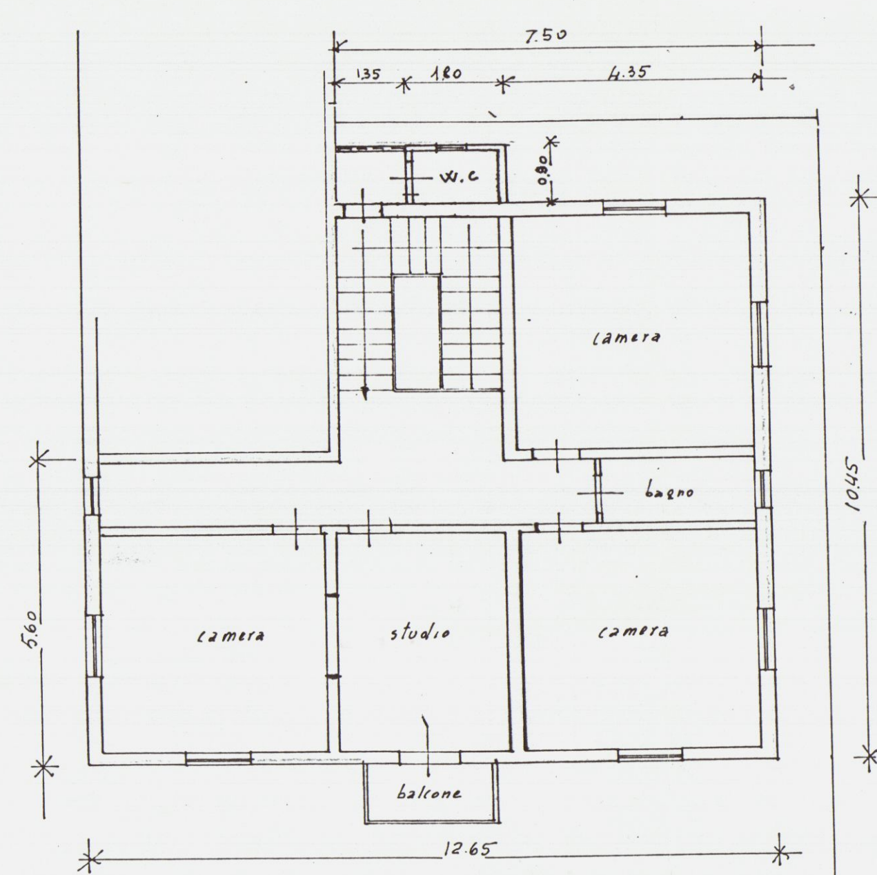
PIANO PRIMO ESISTENTE
