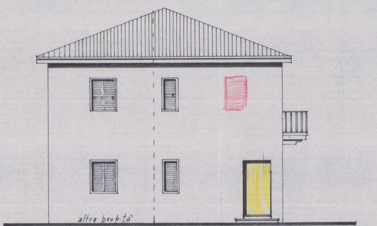
LATO OVEST DA PROGETTO
