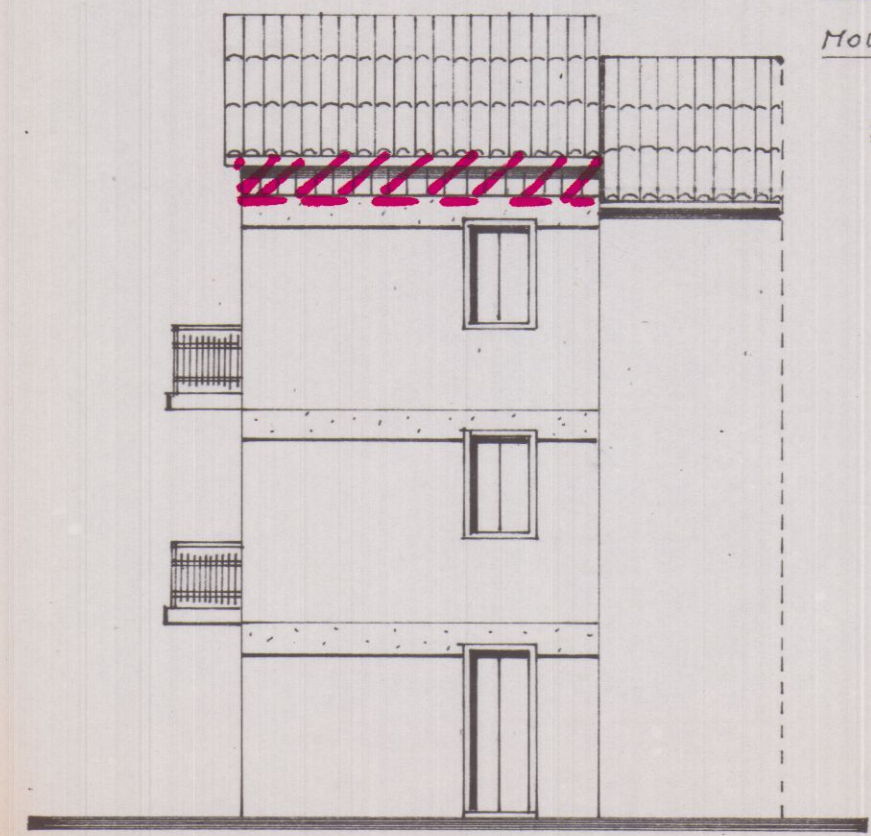
PROSPETTO NORD
