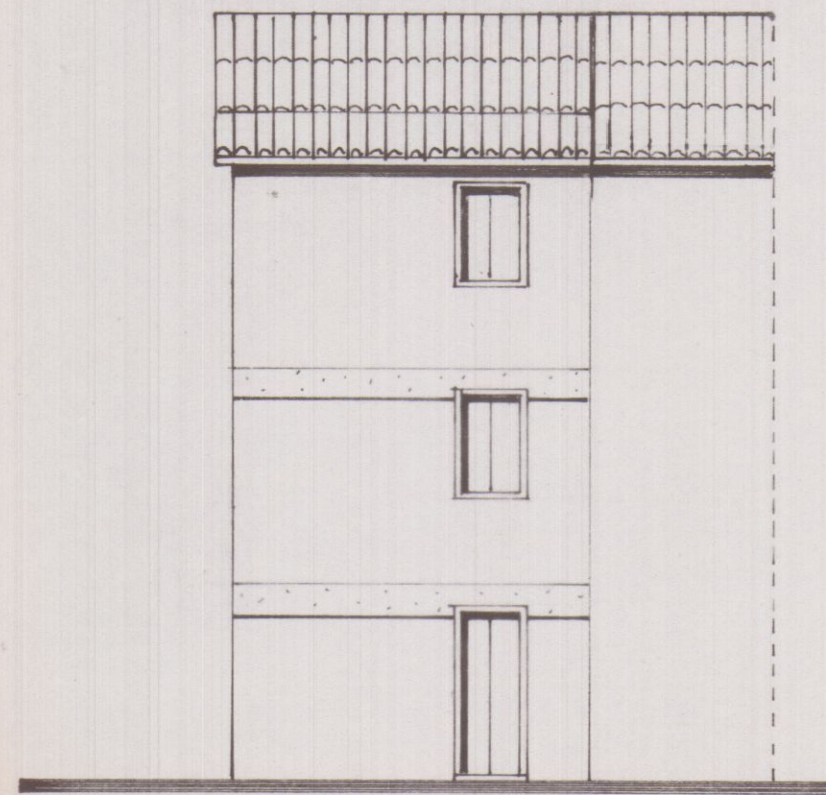
PROSPETTO NORD
