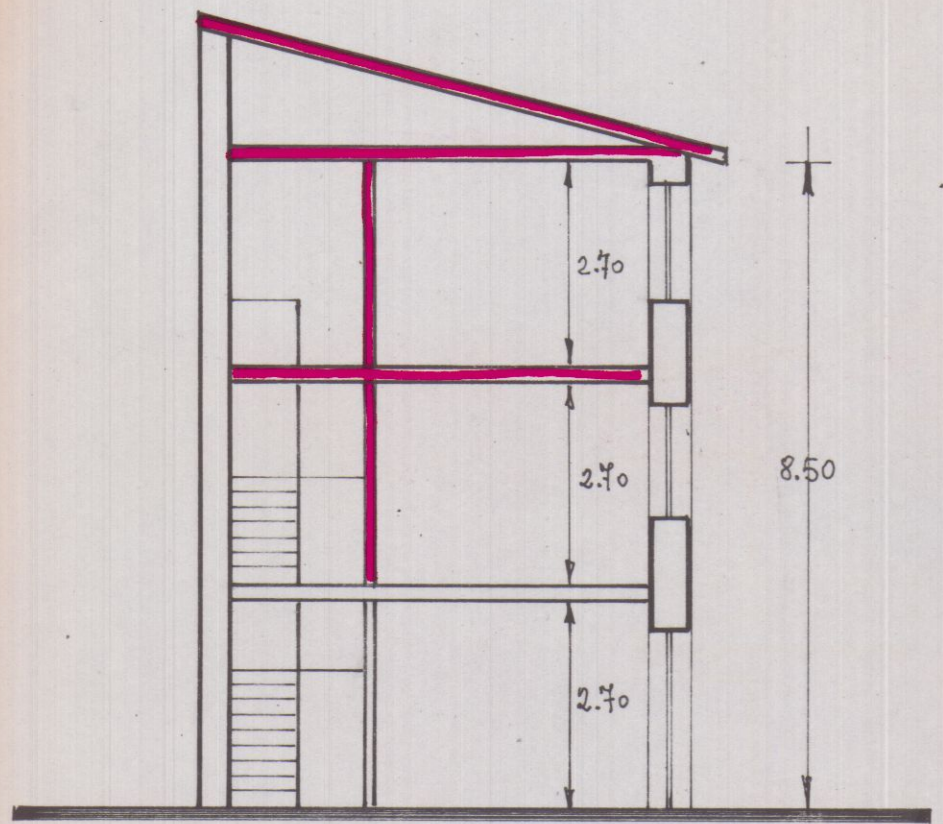
SEZIONE A-A
