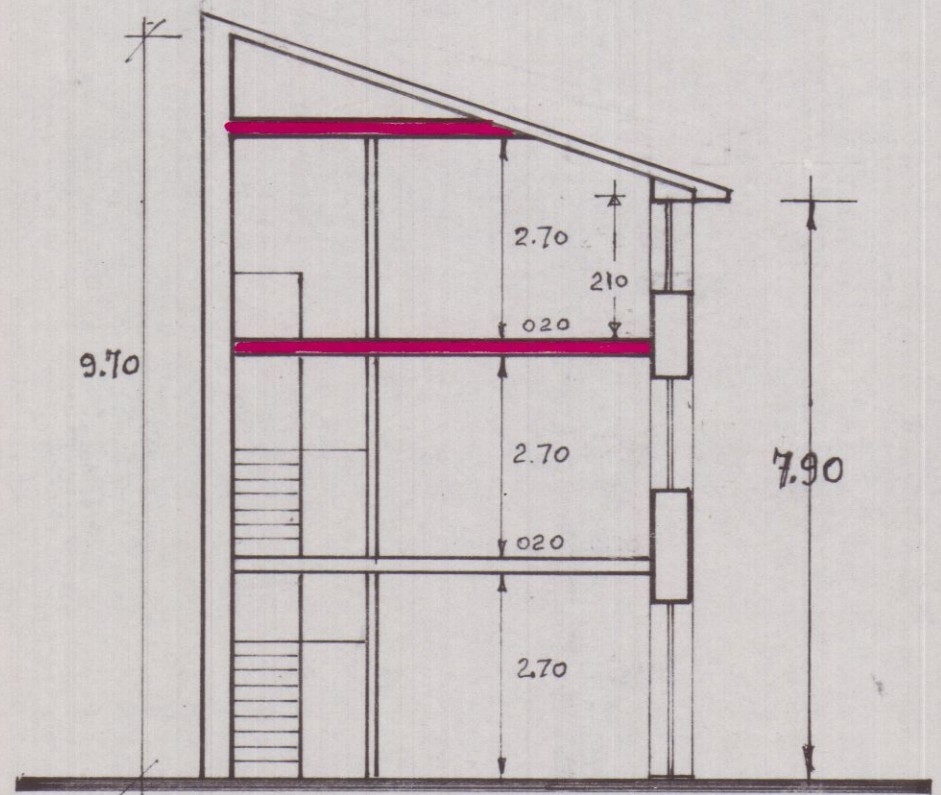
SEZIONE A-A
