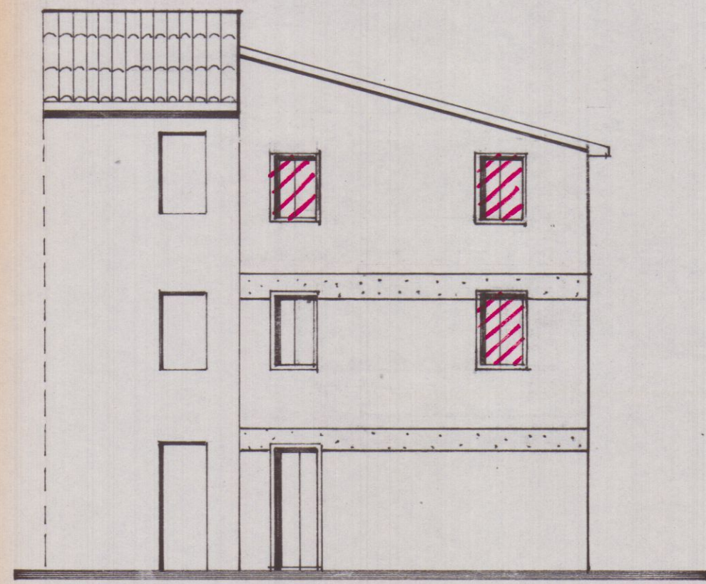
PROSPETTO EST
