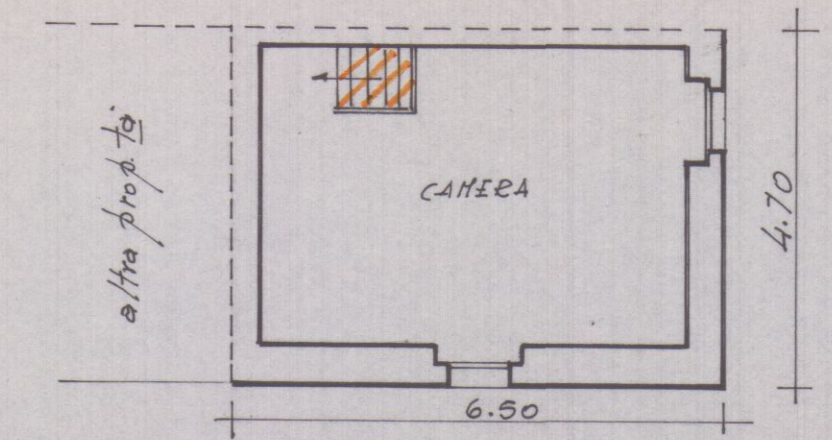
SECONDO PIANO
