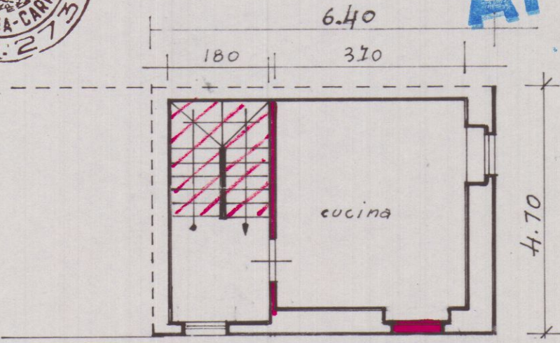
PRIMO PIANO
