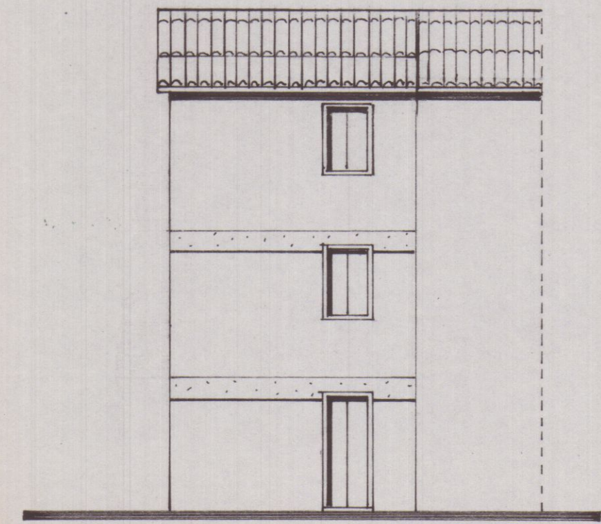
PROSPETTO NORD
