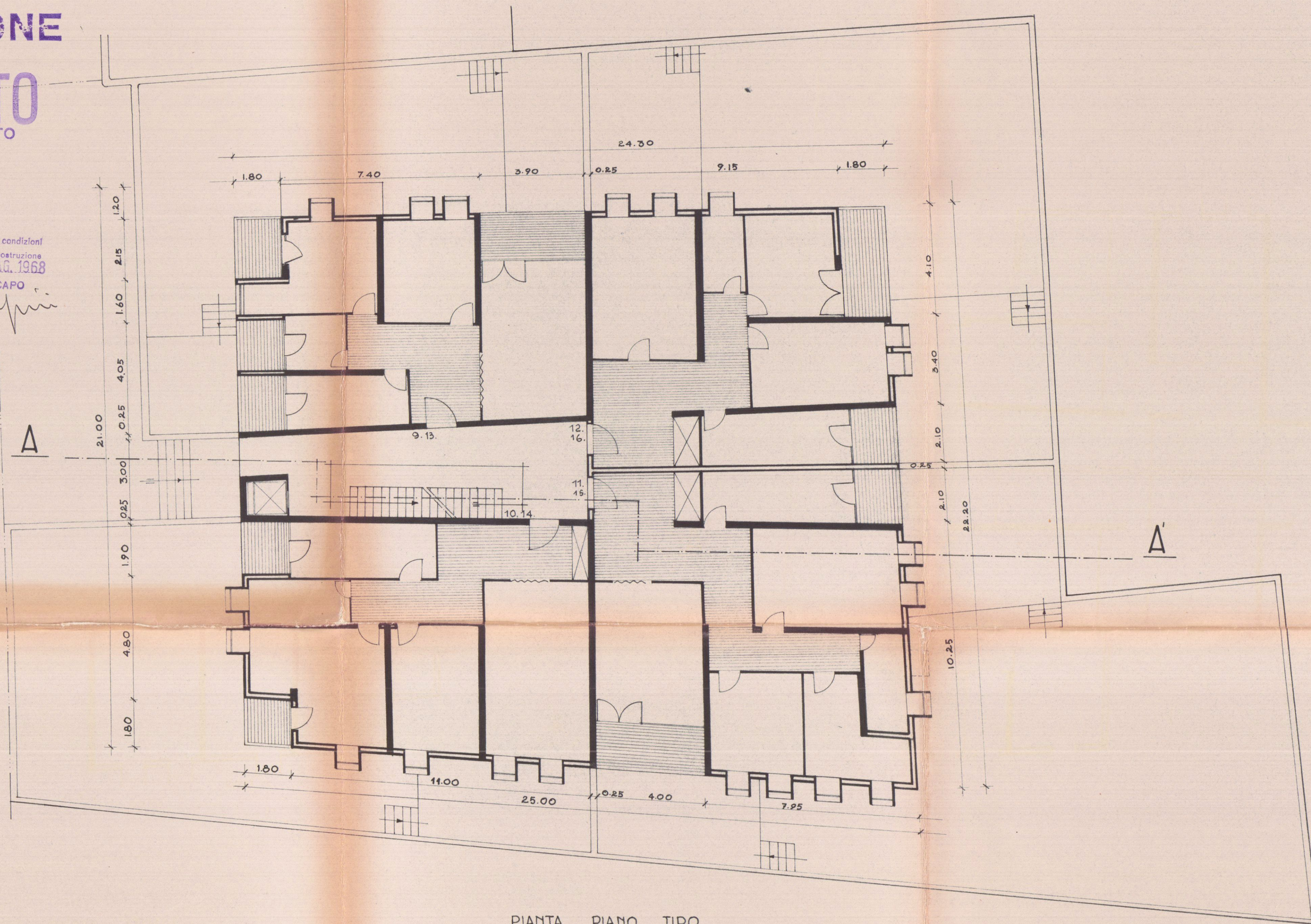
PIANTA PIANO TIPO
