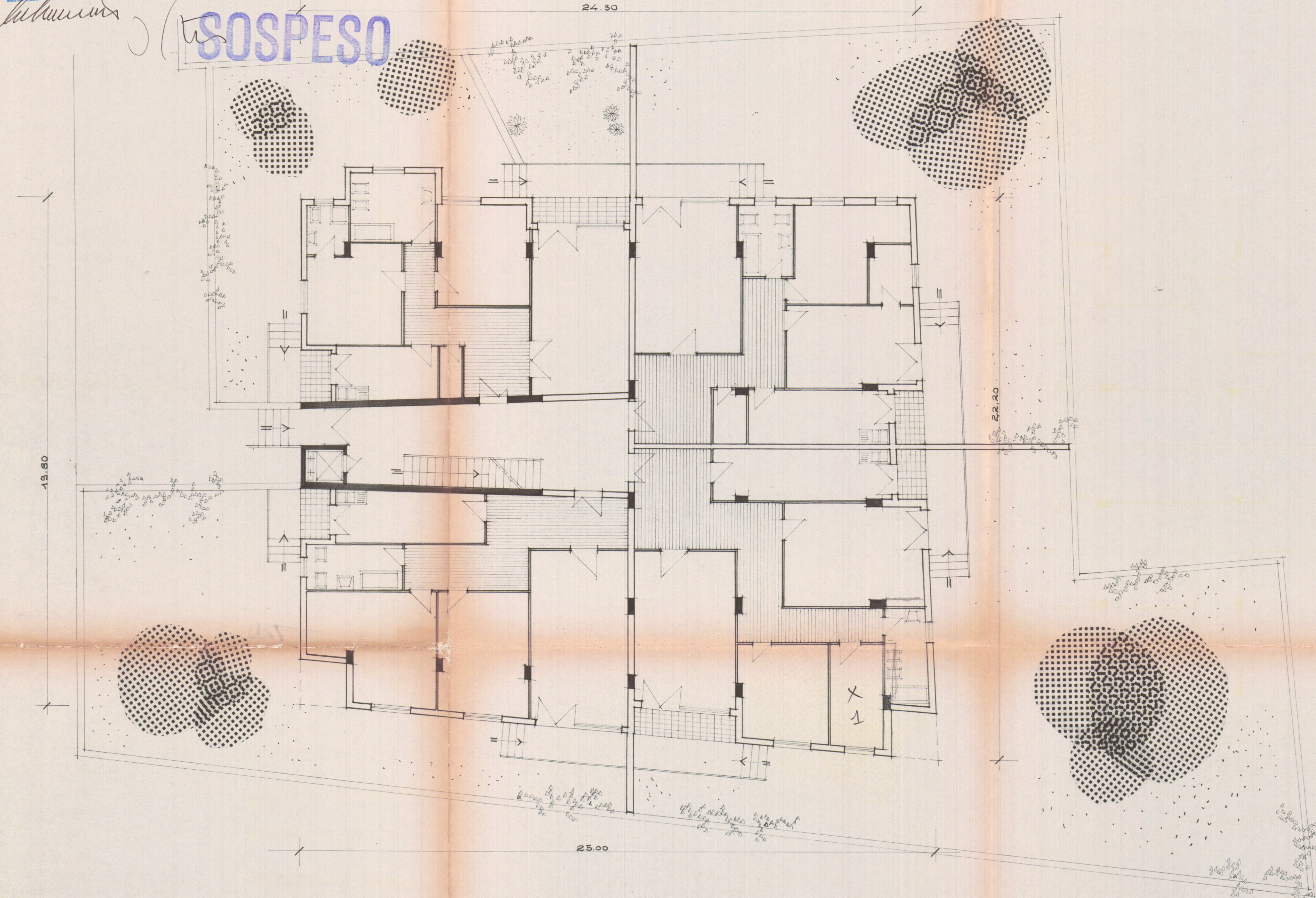
PIANTA PIANO TERRA
