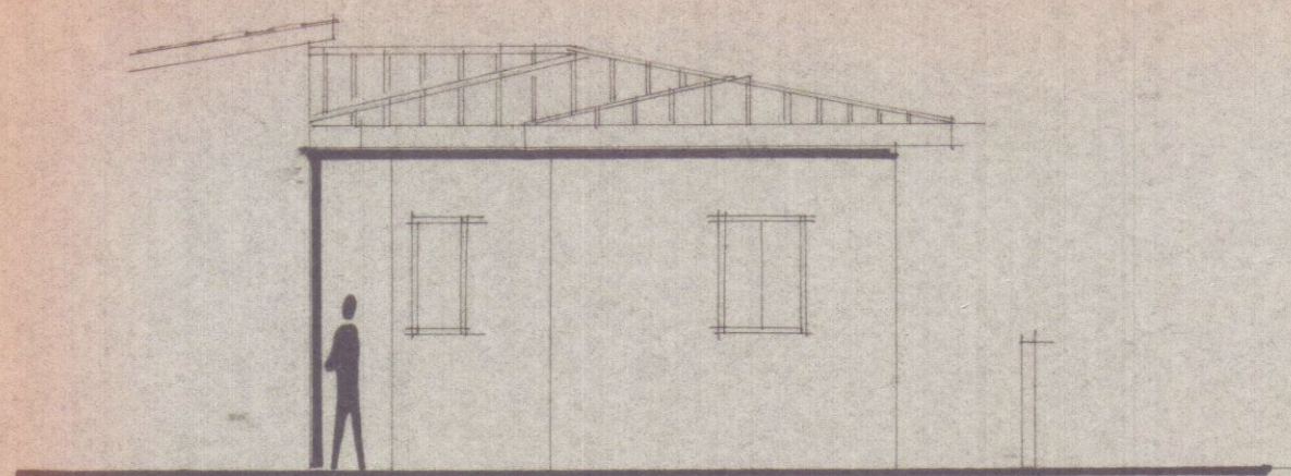
PROSPETTO EST
