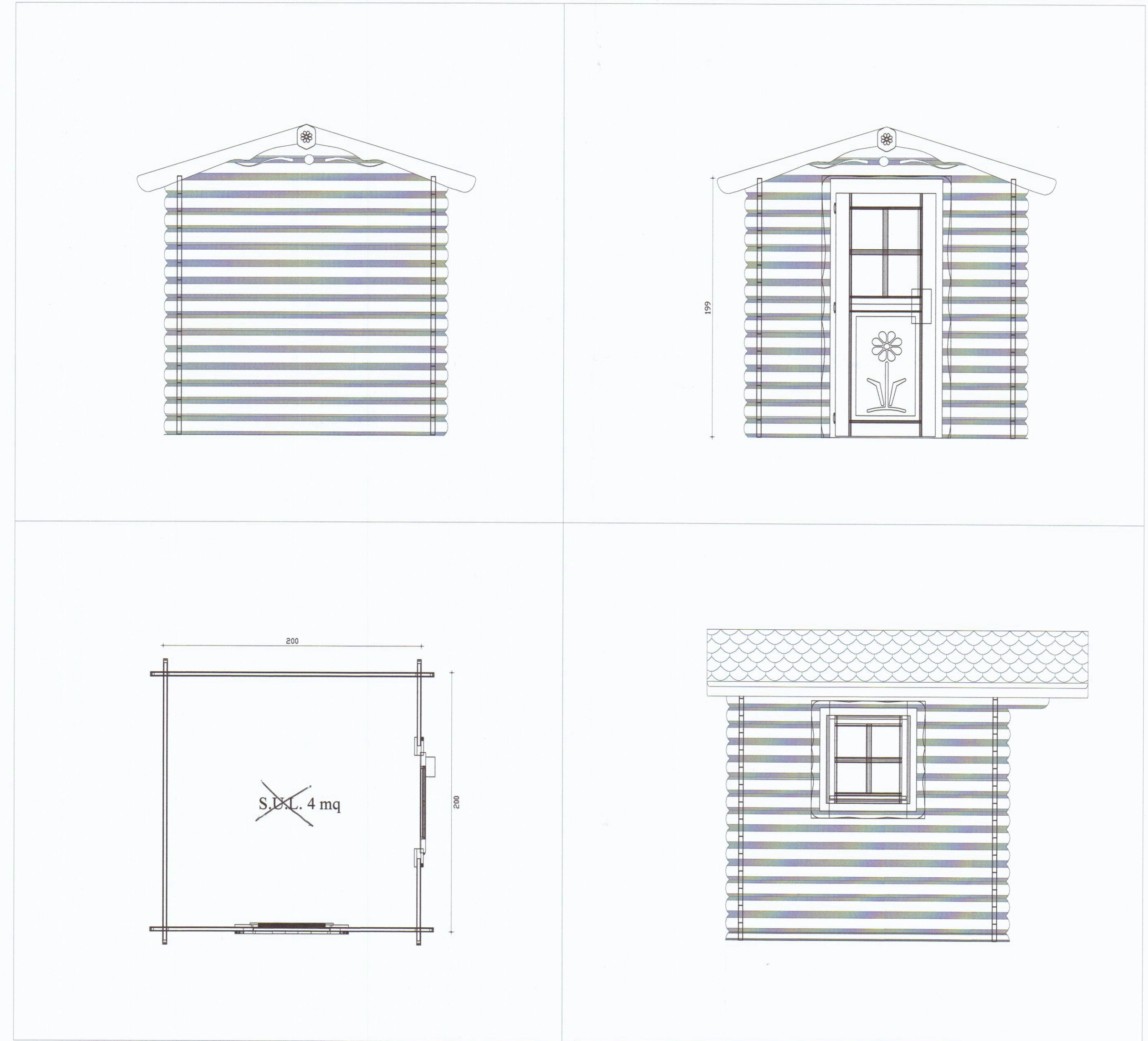
Particolare "A" Casetta in legno - Scala 1:25
