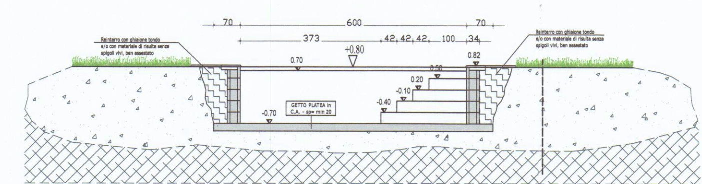
Sezione B - Scala 1:100
