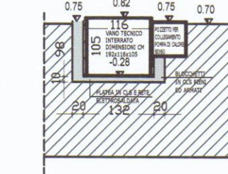
Sezione vano tecnico interrato - Scala 1:100 Particolare B
