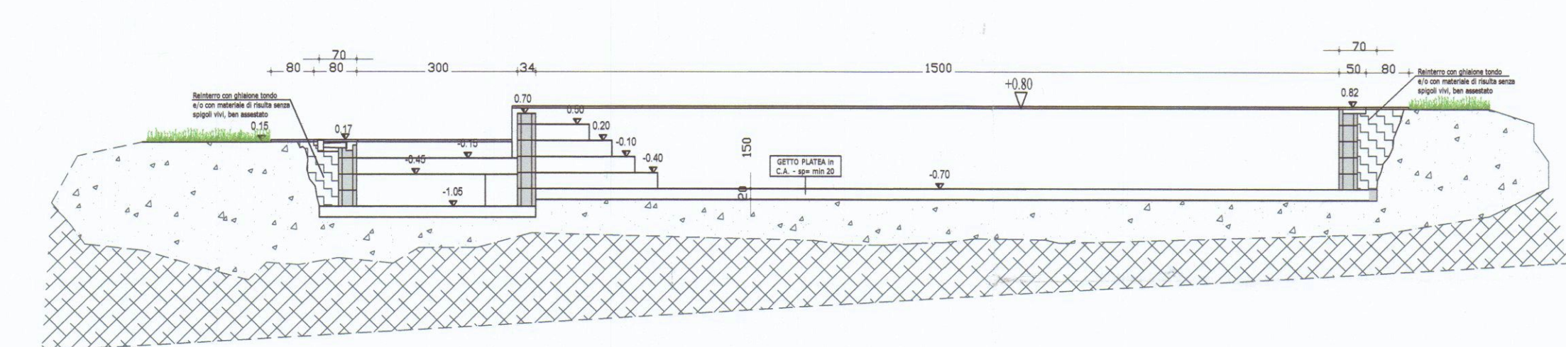
Sezione A - Scala 1:100
