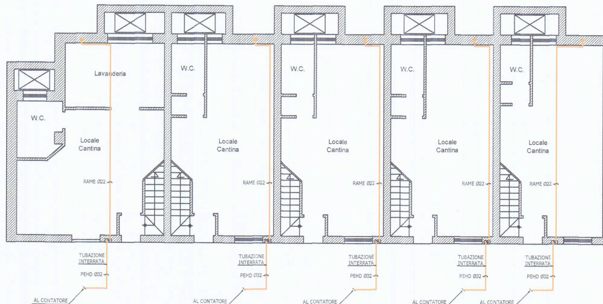
Pianta piano seminterrato
