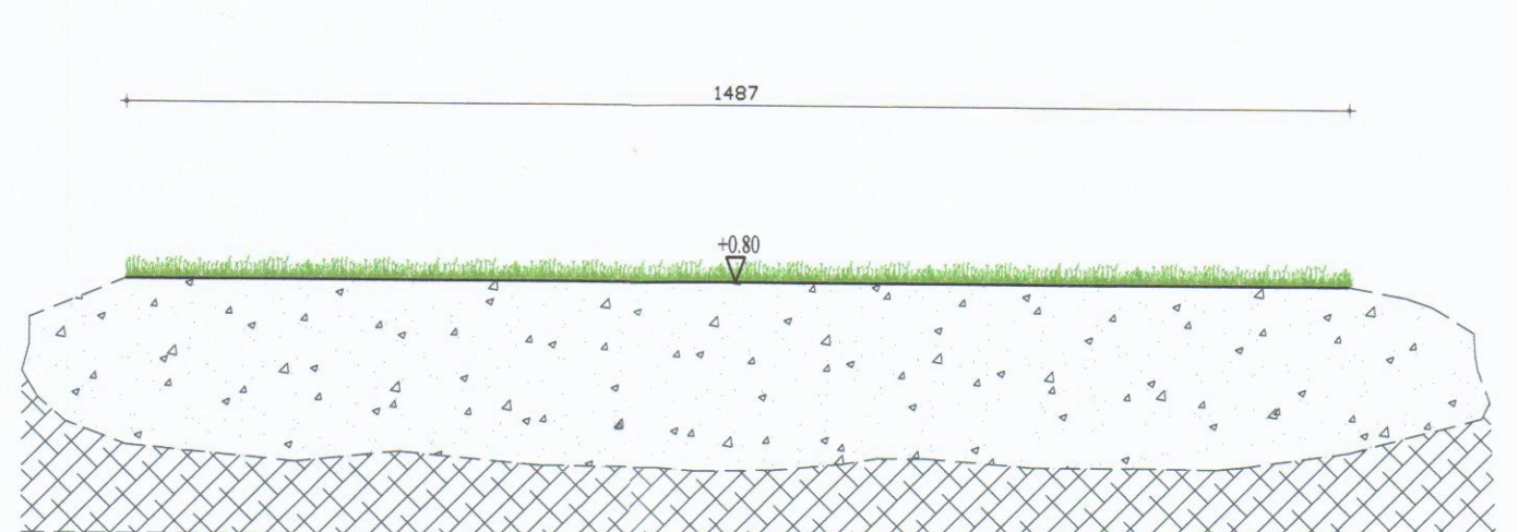
Sezione B - Scala 1:100
