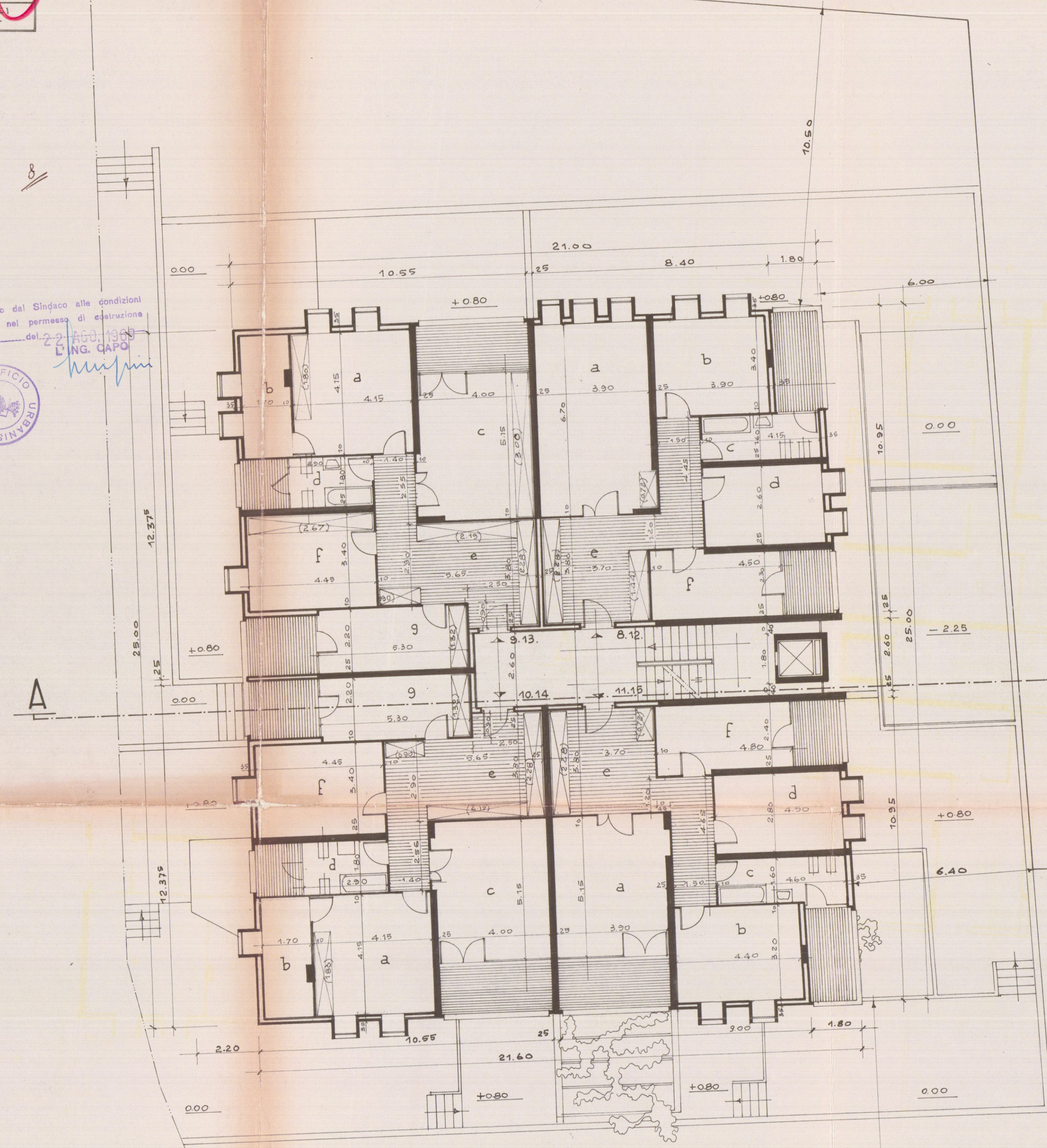
PIANTA PIANO TIPO
