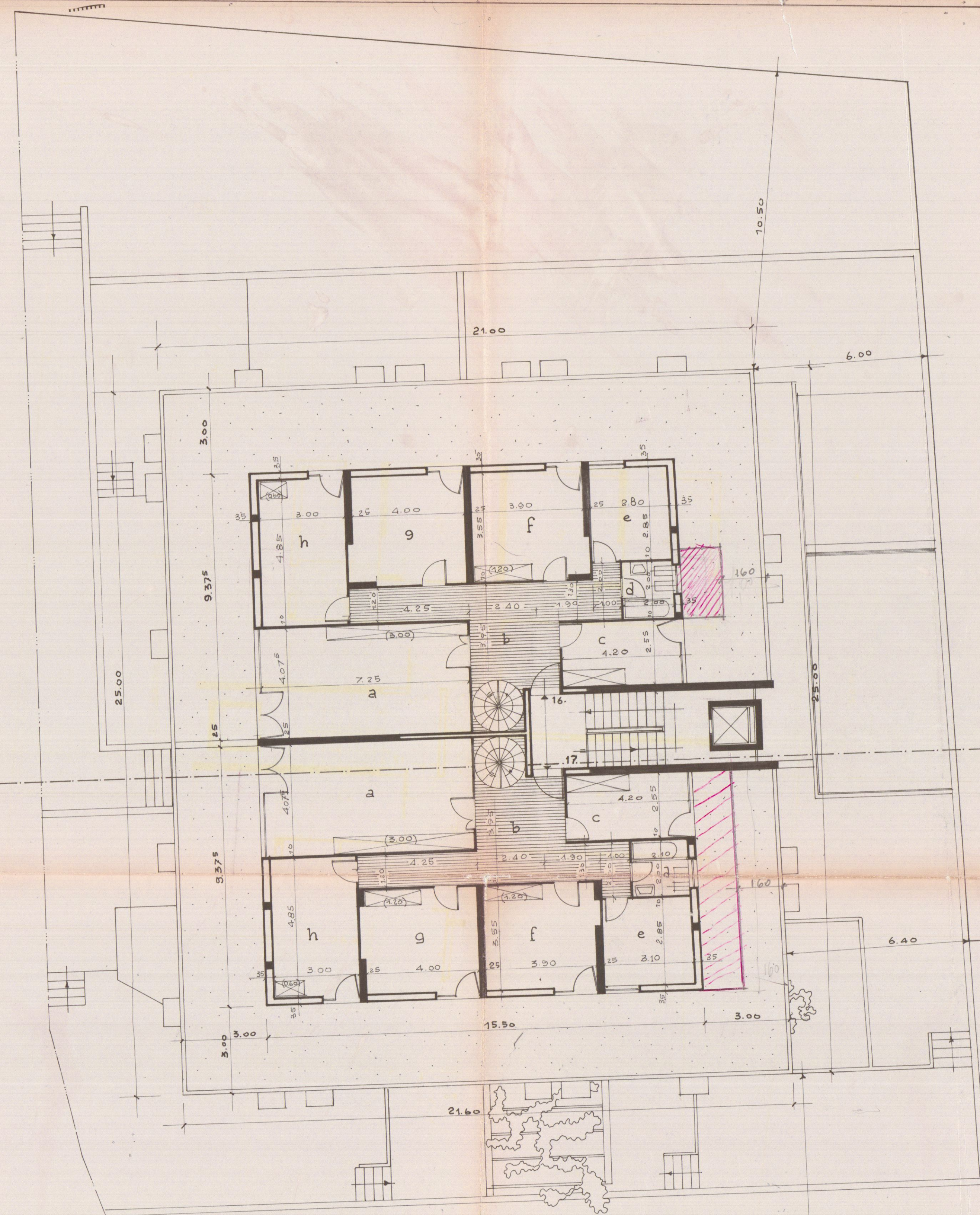
PIANTA PIANO ATTICO
