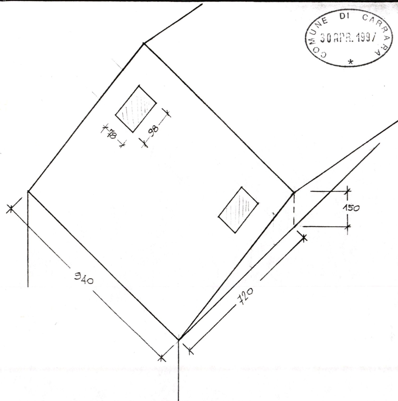
SCHEMA INSTALLAZIONE FINESTRE Scala 1:100
