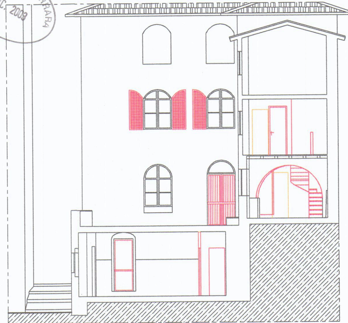
Sezione D:D
