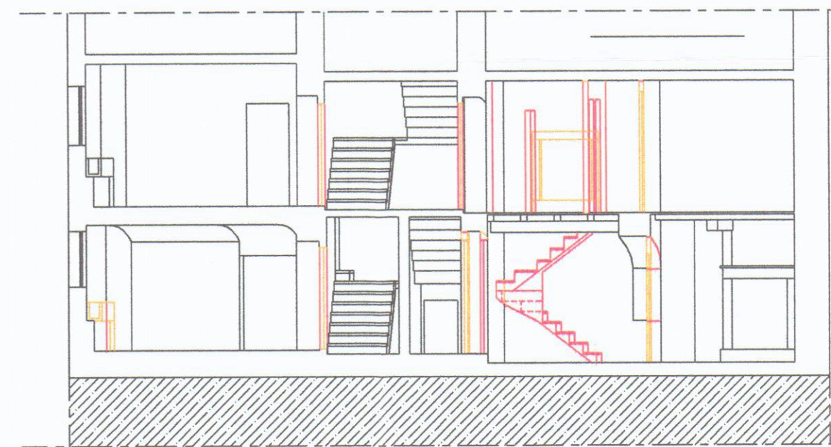
Sezione C:C
