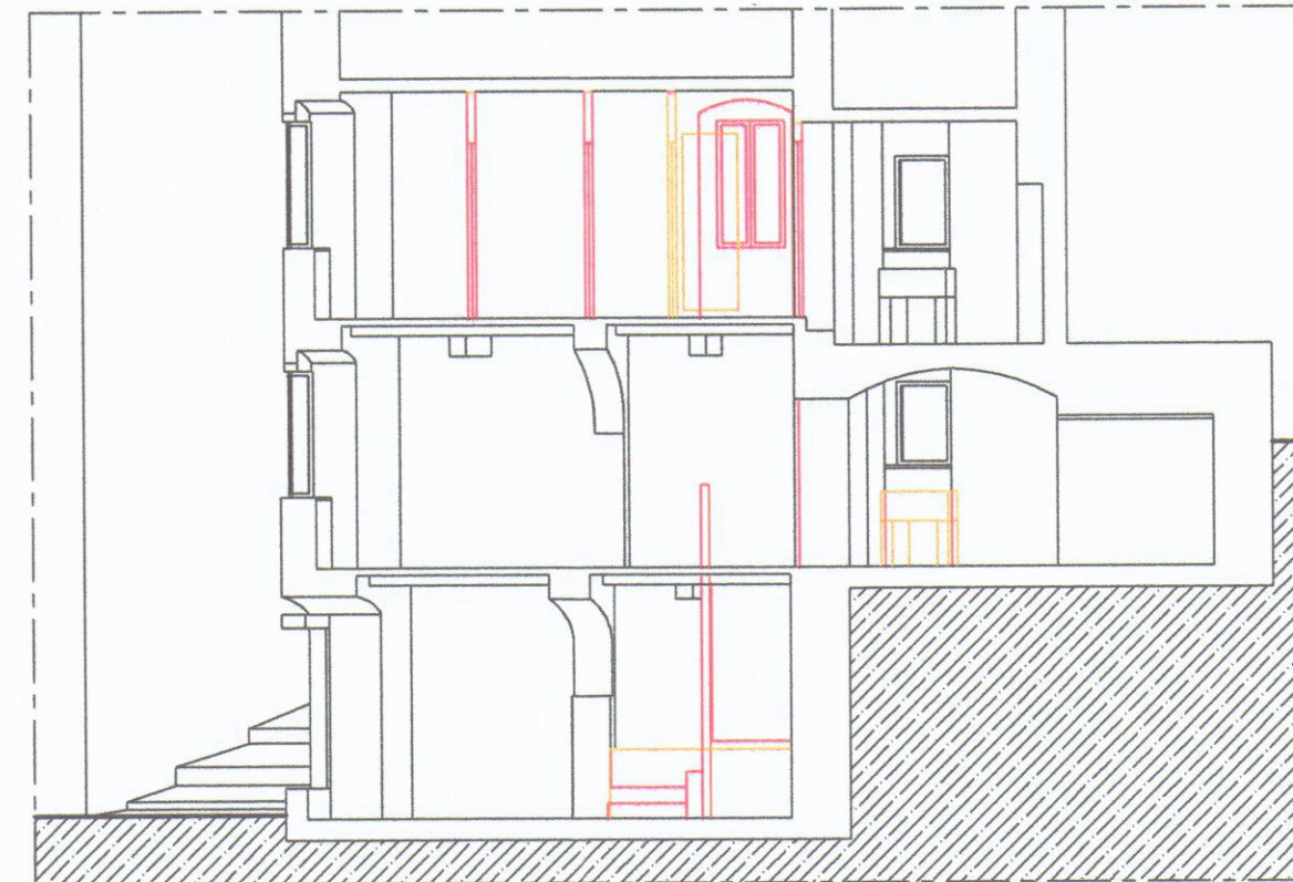
Sezione B:B
