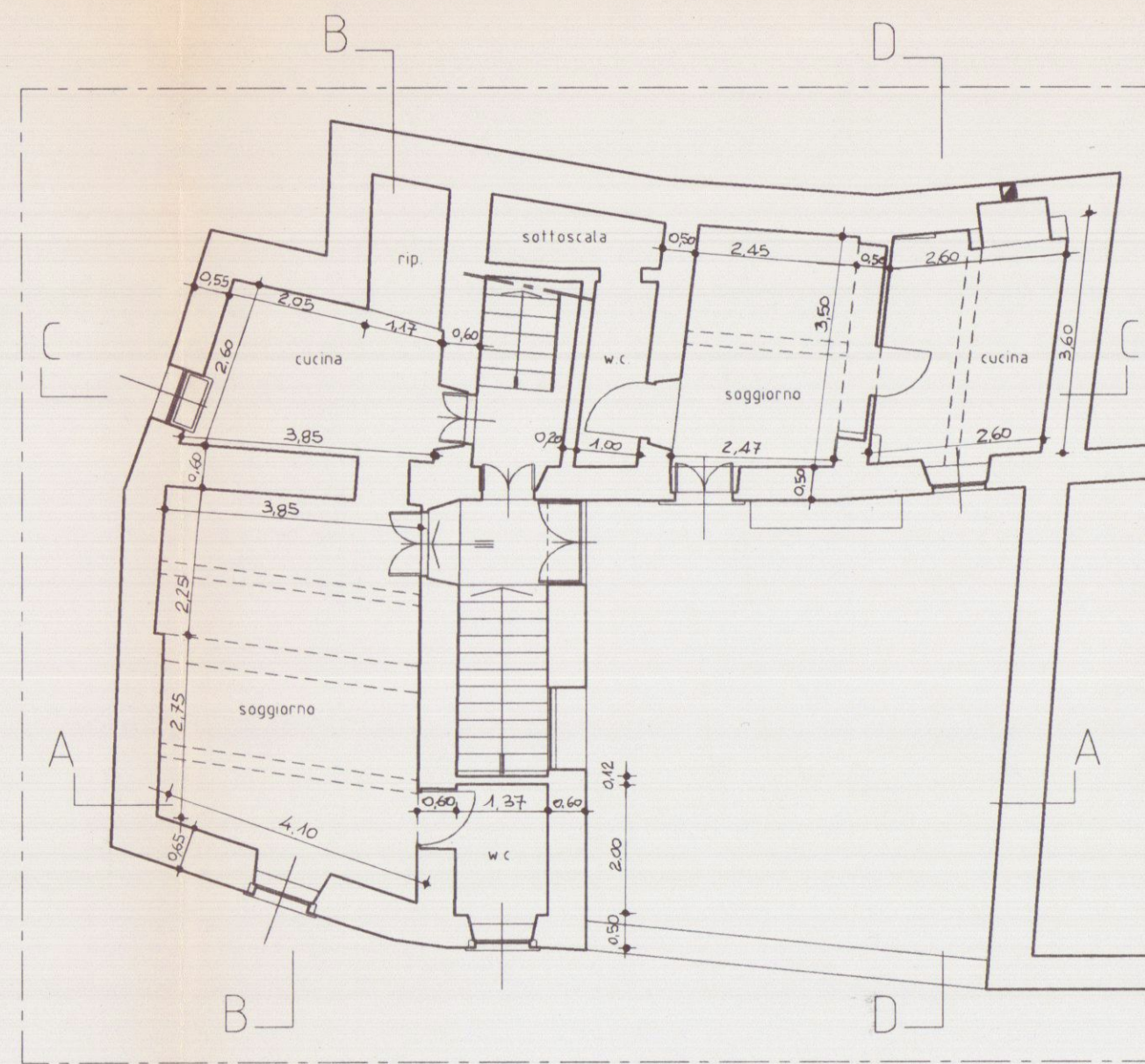
Piano Primo
