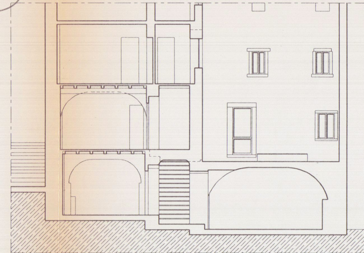
Sezione A:A
