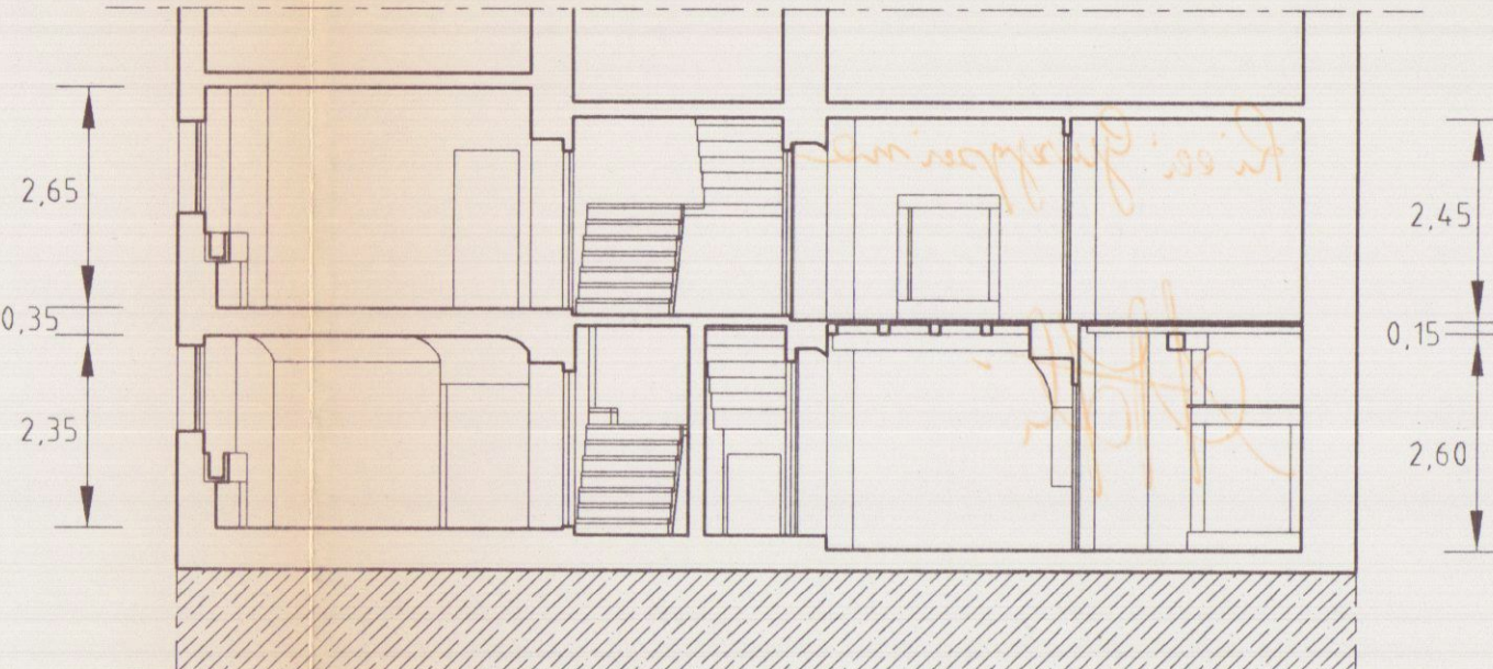
Sezione C:C
