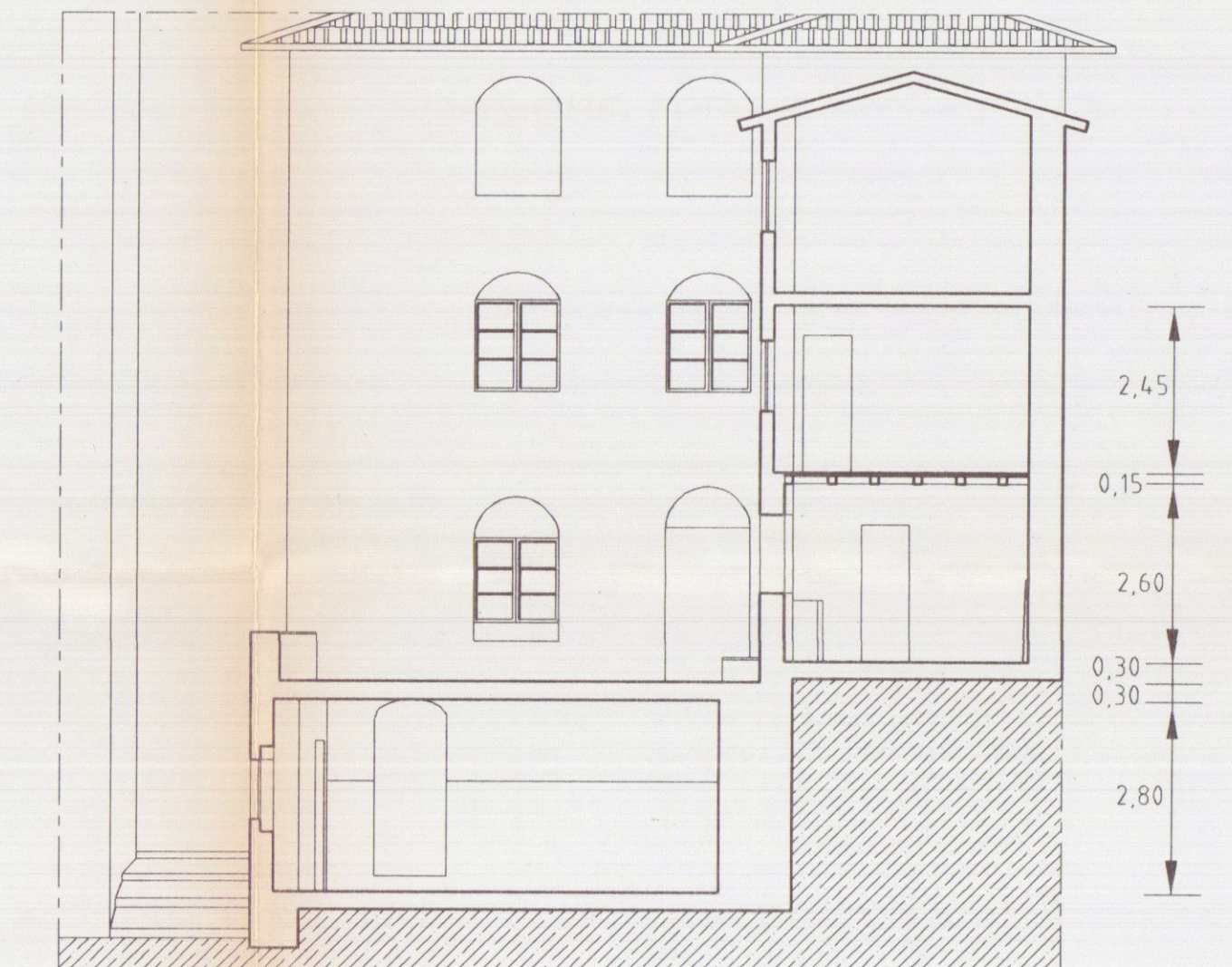
Sezione D:D
