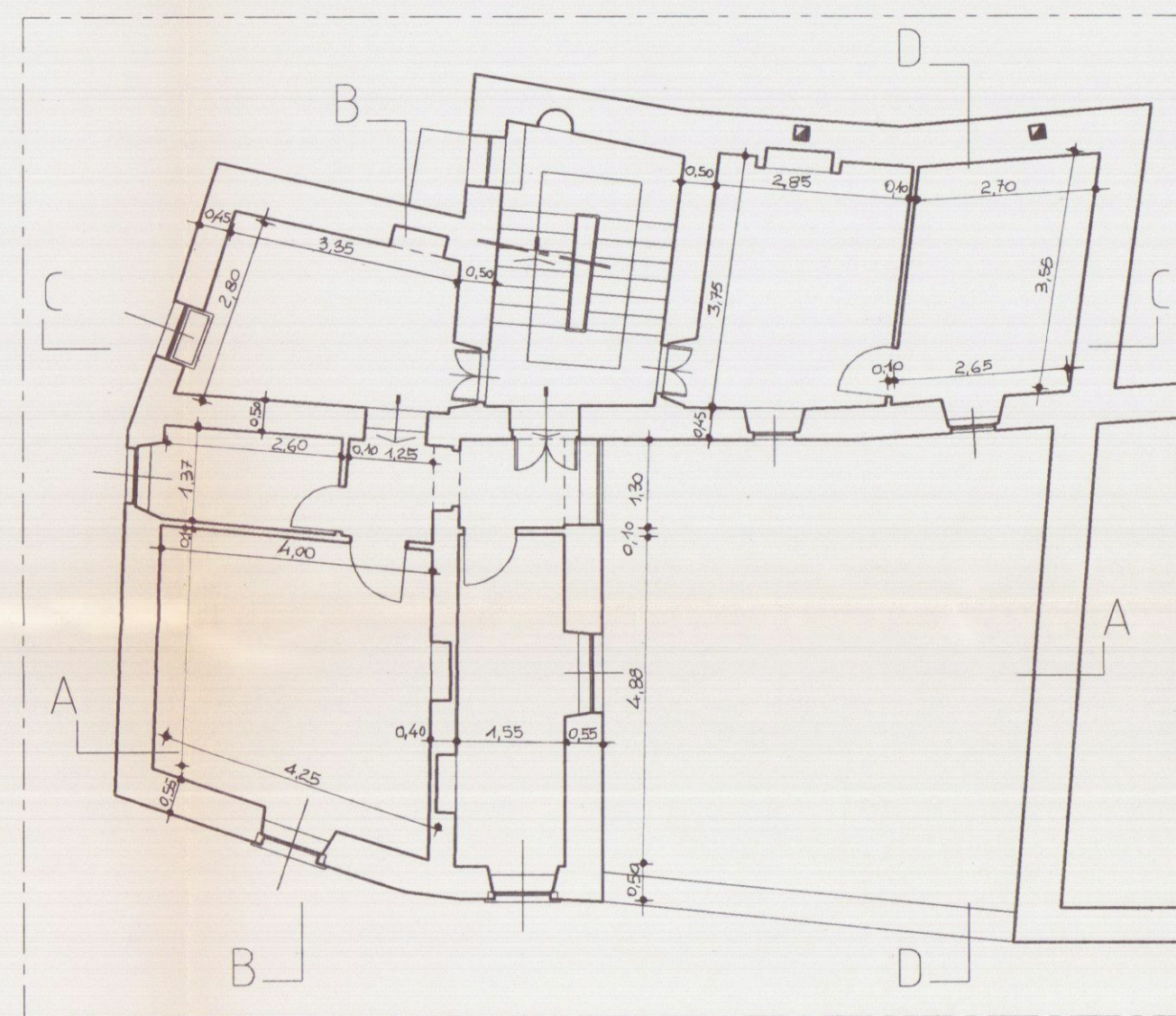
Piano Secondo
