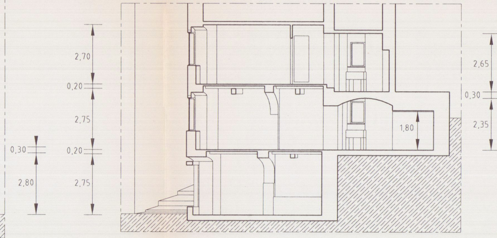
Sezione B:B
