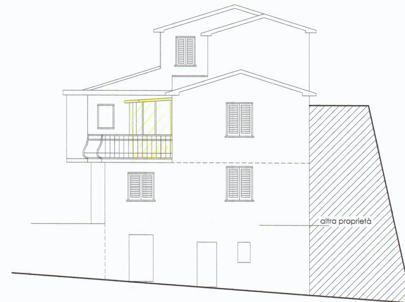
PROSPETTO SUD
