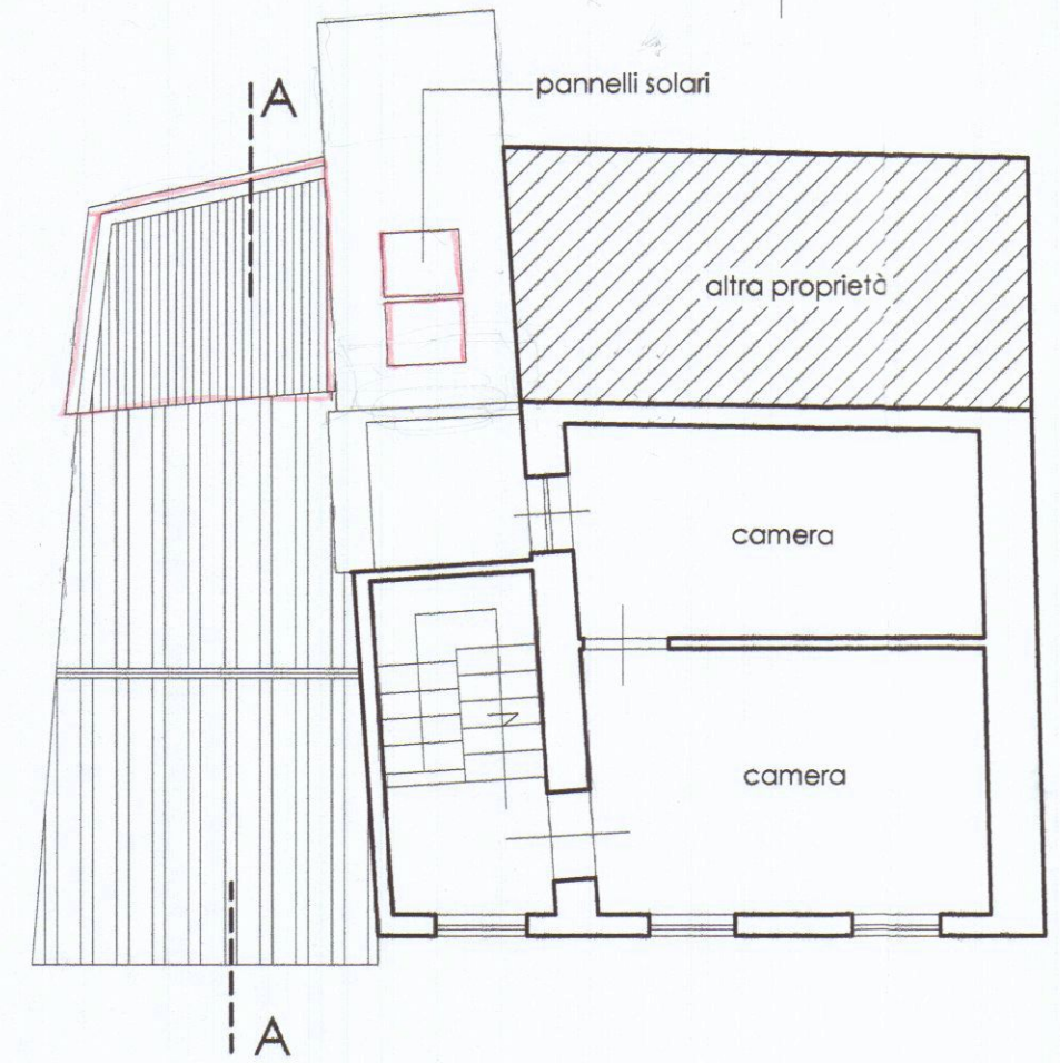
PIANO SECONDO
