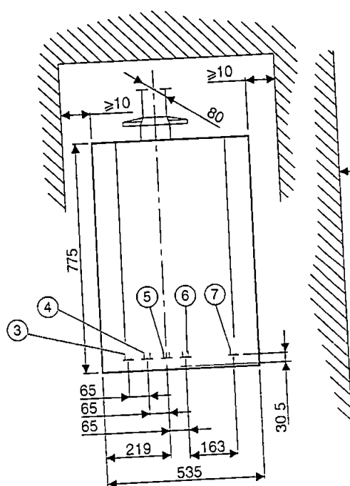
Fig 3 vista frontale
