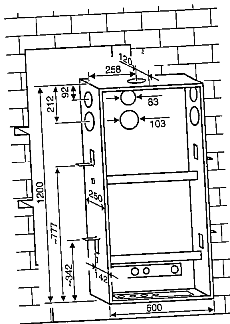
Fig 1 vista frontale
