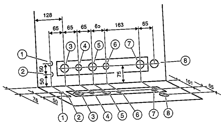
Fig 2 vista allacciamenti elettrici ed idraulici
