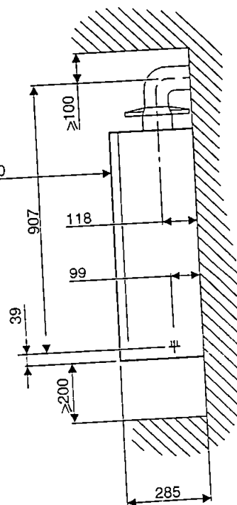
Fig 4 vista laterale
