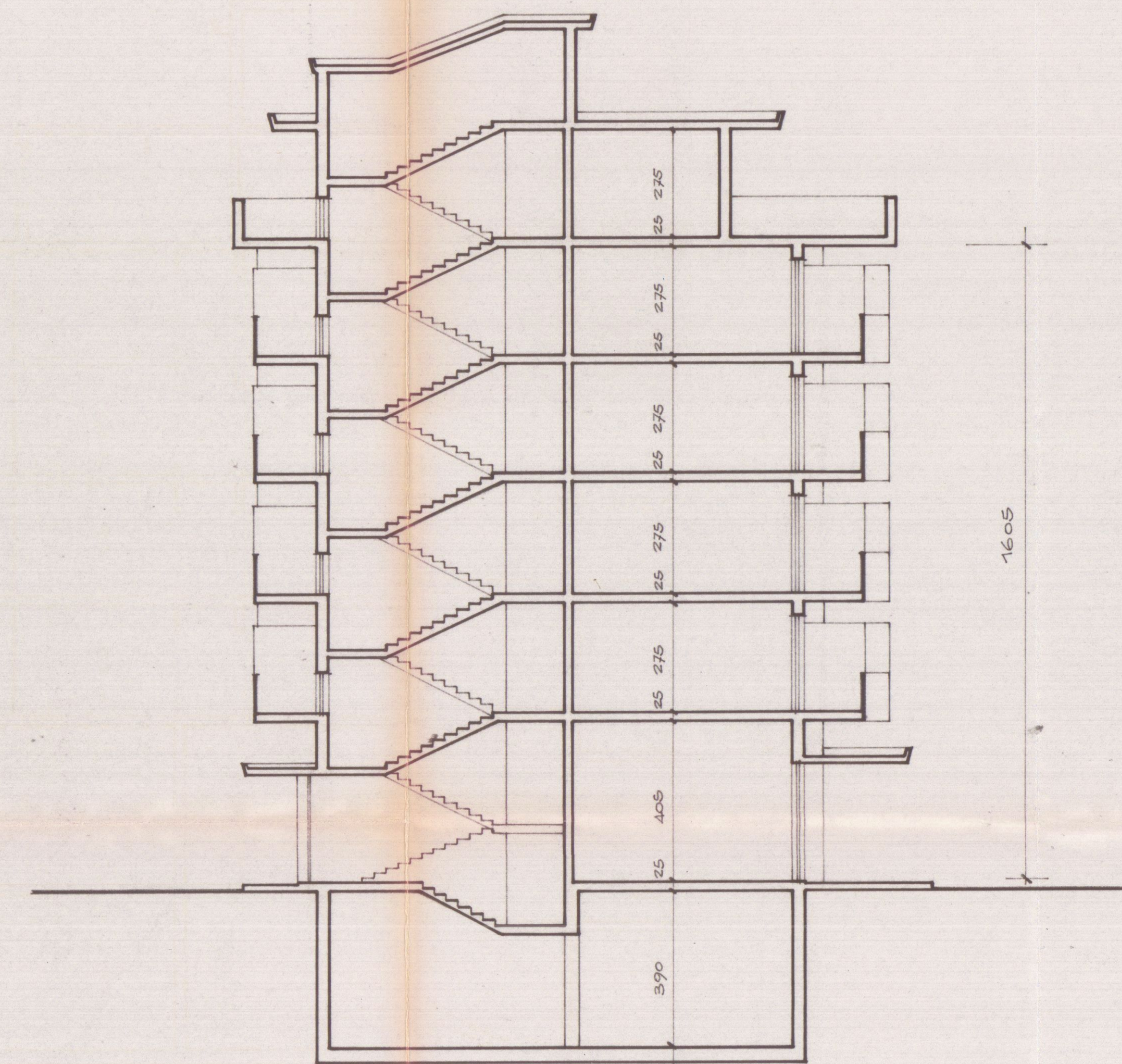
SEZIONE TRASVERSALE
