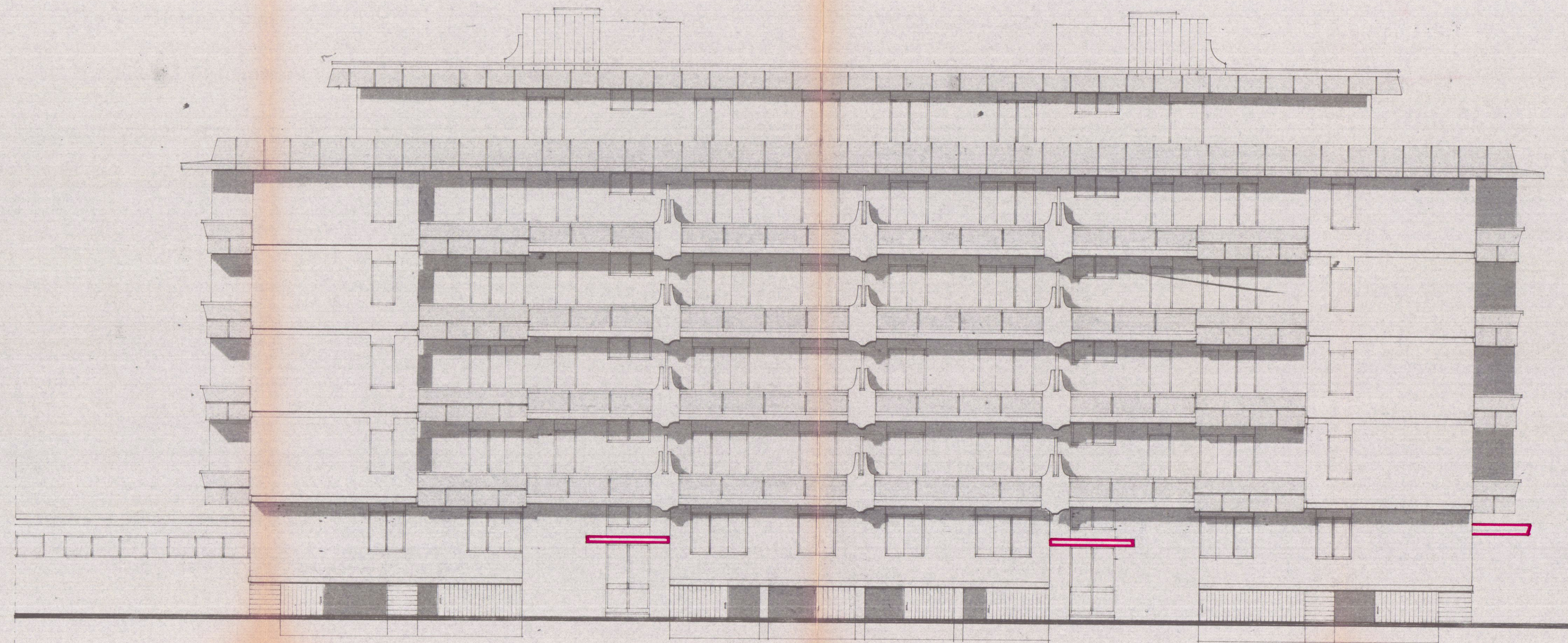
PROSPETTO OVEST
