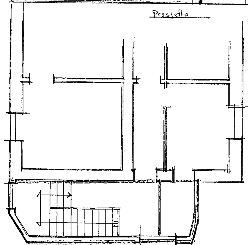
Pianta P. 1°
