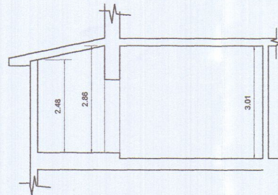
SEZIONE A-A
