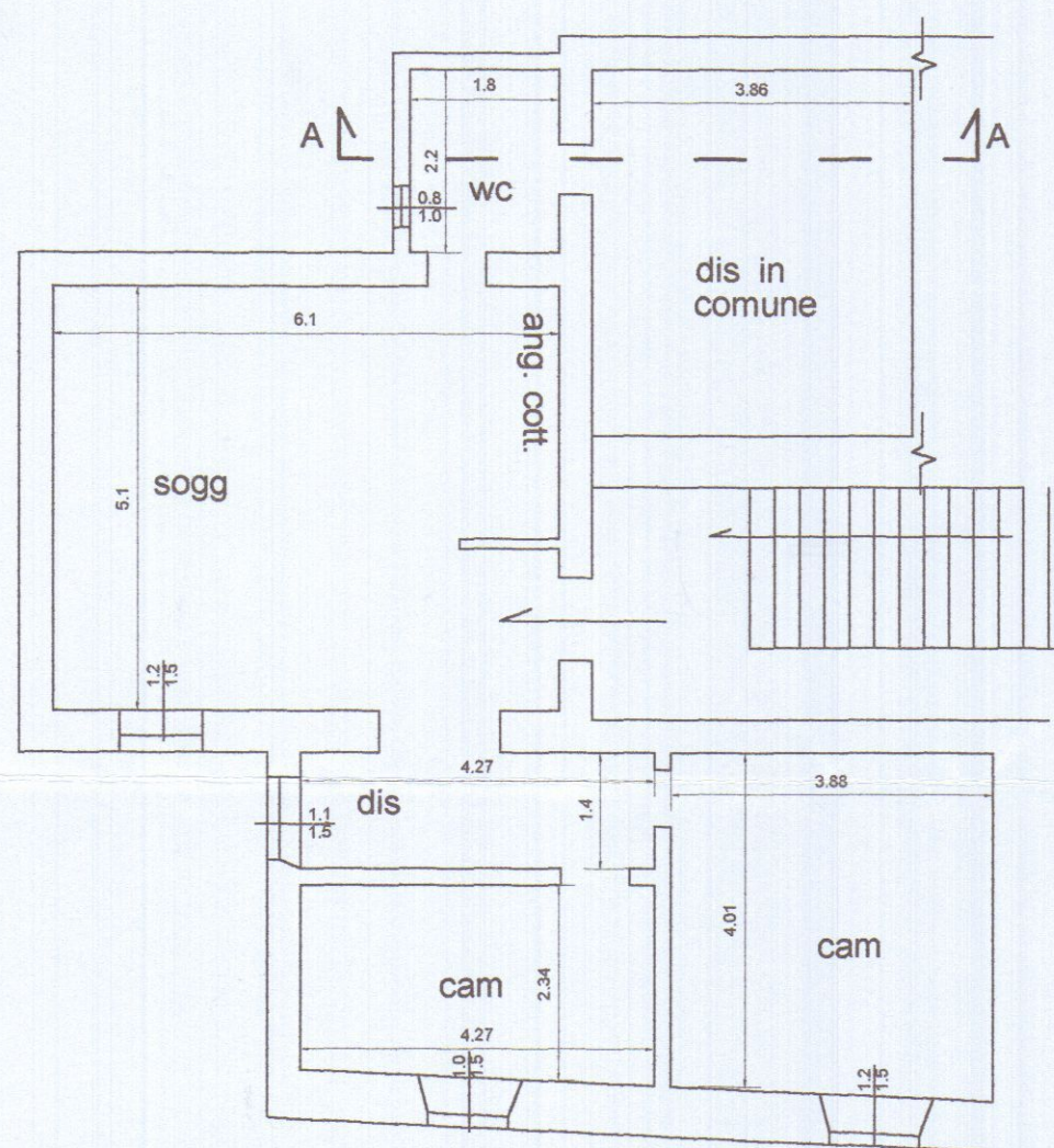
PIANO SECONDO
