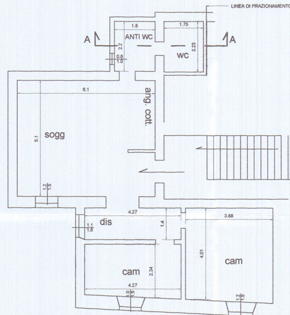
PIANO SECONDO
