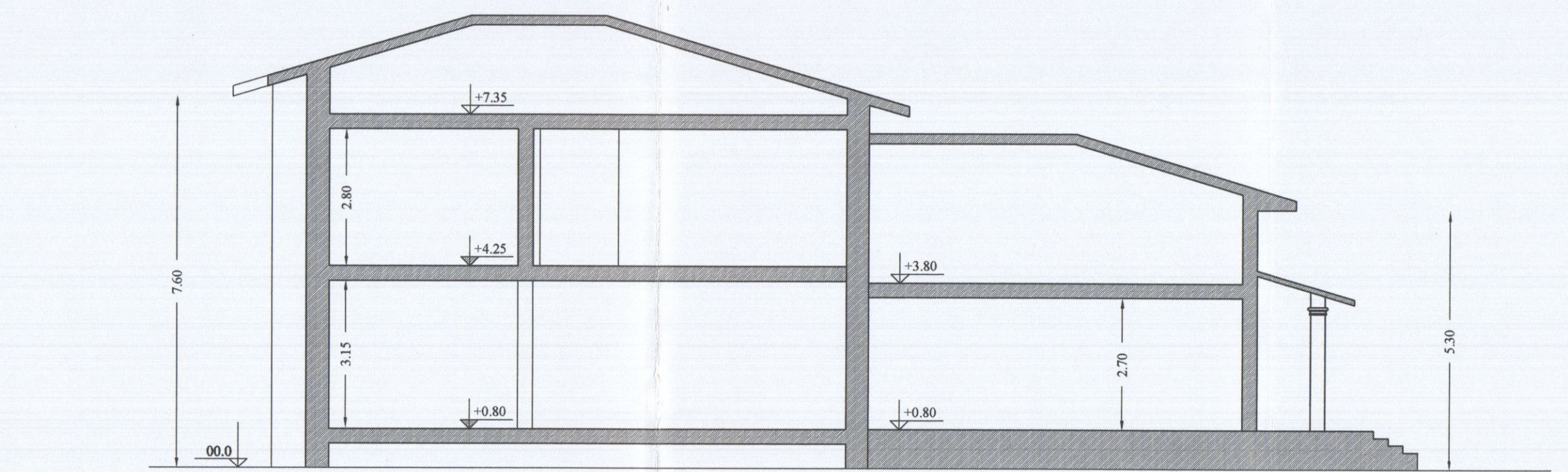
sezione A-A
