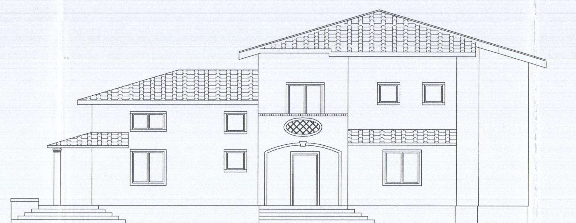
PROSPETTO EST DI PROGETTO
