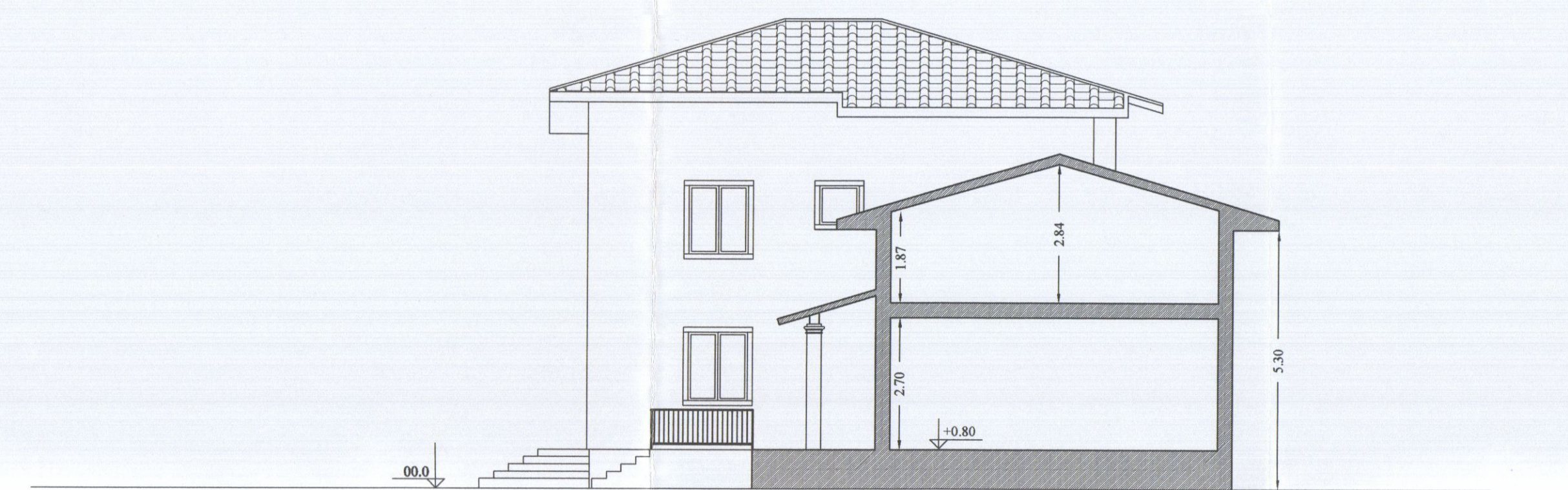
sezione B-B
